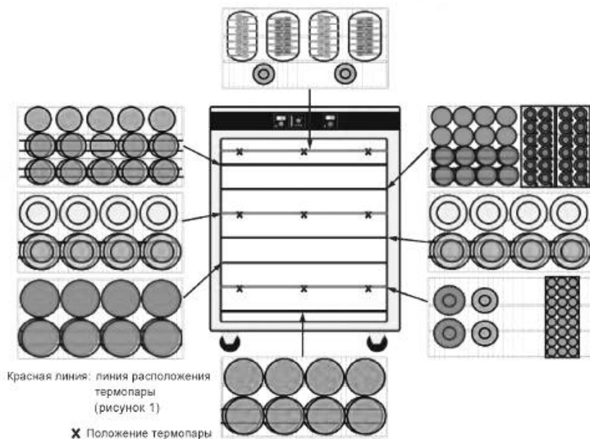
Рисунок G.1 — Положение термодпары на верхней, средней и нижней проводной пластине
