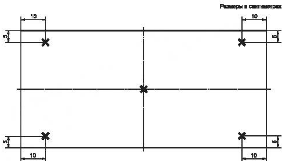
Рисунок G.1 — Положение термодпары на верхней, средней и нижней проводной пластине
