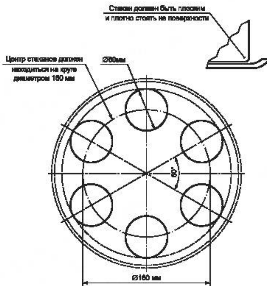
Рисунок 1 — Расположение стаканов на поворотном диске микроволновой печи
