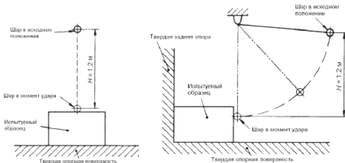
Рисунок 101 – Испытания на удар с помощью стального шара
