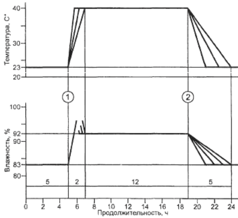
Рисунок 102 – График температуры и влажности
