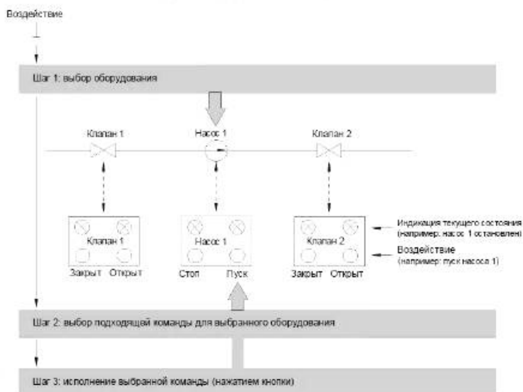
Рисунок 1 — Трехшаговая последовательность пуска для однофункционального применения
