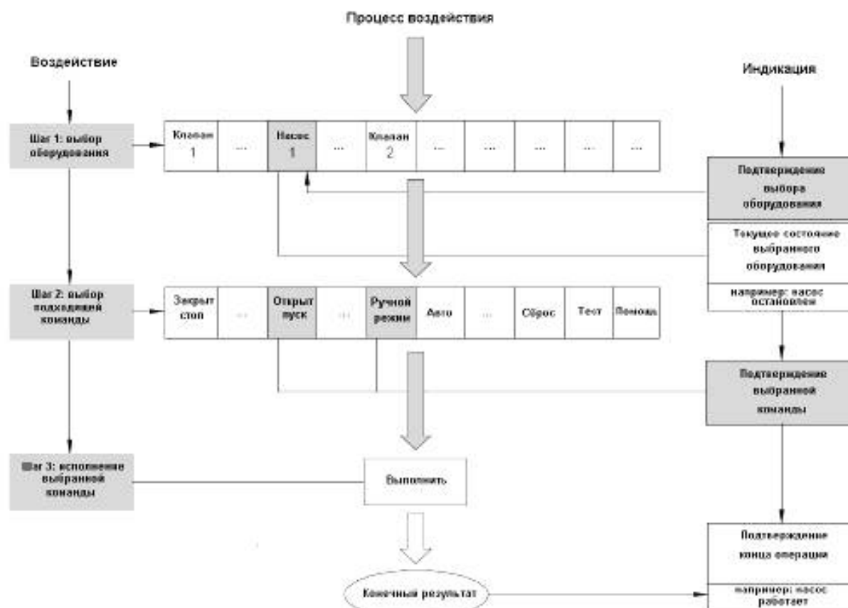
Рисунок 2 — Трехшаговая последовательность пуска для многофункционального применения
