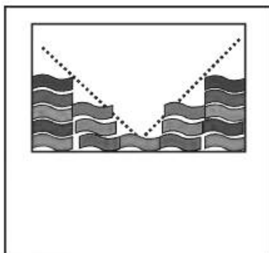
Рисунок J.5 — Три площади загрузки
