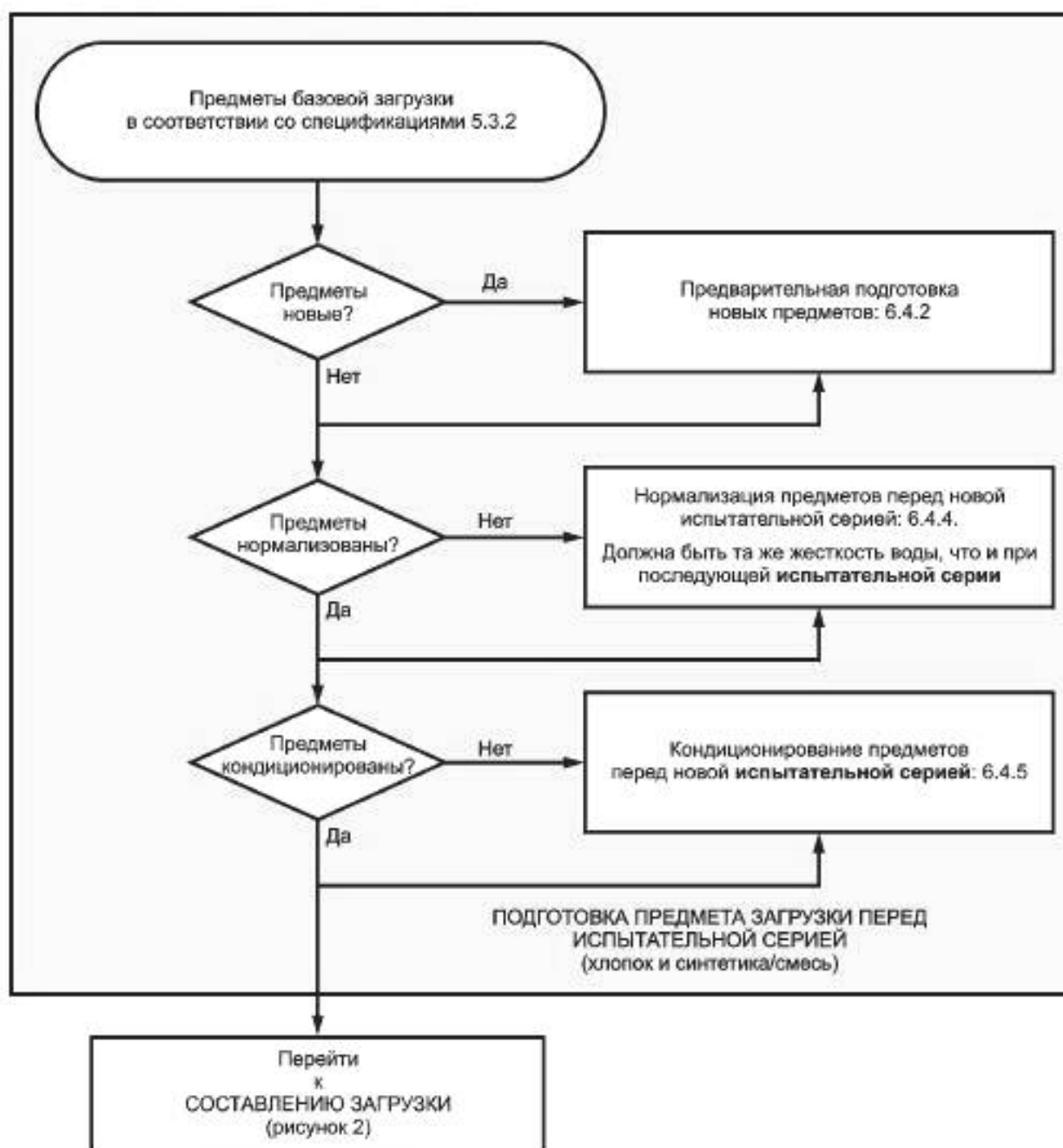
Рисунок 1 — Подготовка предметов загрузки перед испытательной последовательностью
