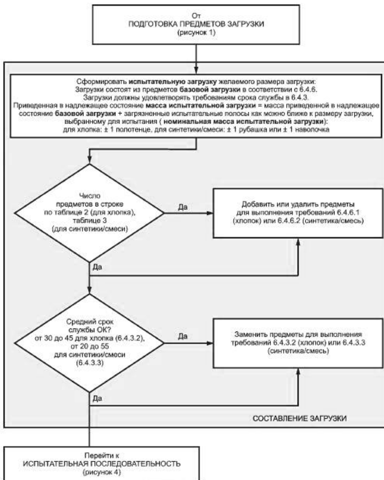
Рисунок 2 — Составление загрузки и требования к сроку службы
