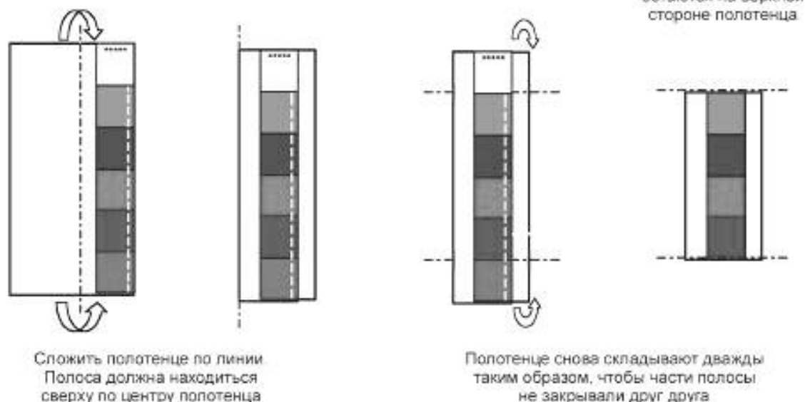
Рисунок Н.1 — Складывание полотенца с прикрепленной загрязненной испытательной полосой
