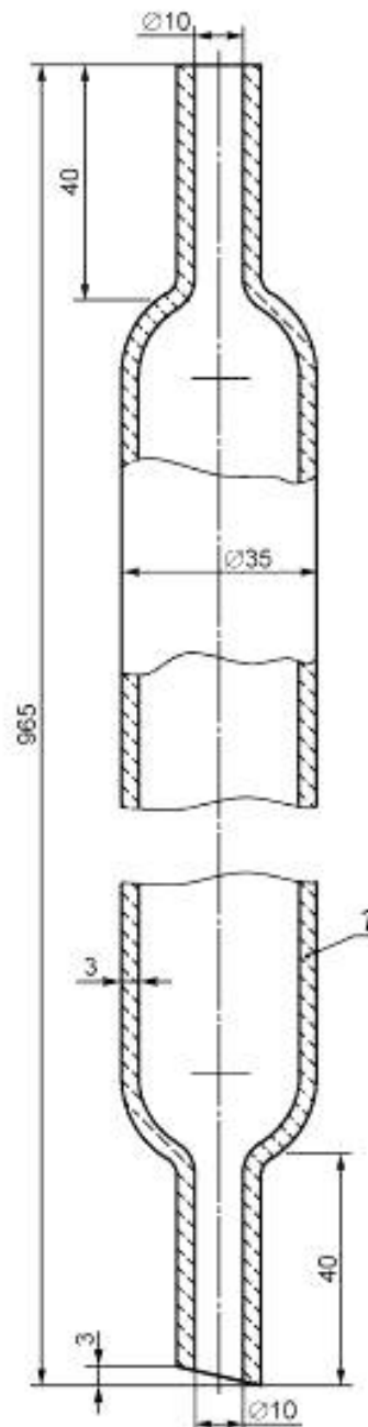
1 — стеклянная трубка, зауженная с обоих концов
