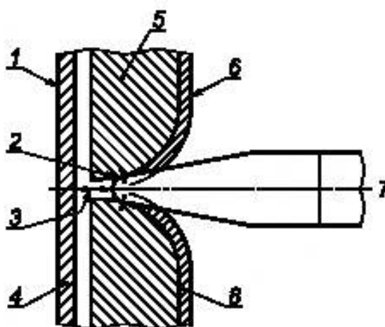
1 — внутренняя часть; 2 — точка, от которой измеряют пути утечки; 3 — зазор; 4 — доступная часть, прикосновение к которой представляет опасность; 5 — покрытие; 6 — наружная часть; 7 — испытательный палец; 8 — фиктивный проводящий слой
