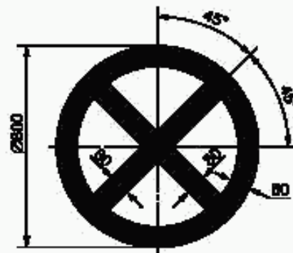
Рисунок 2 — Условное обозначение подруливающего устройства
