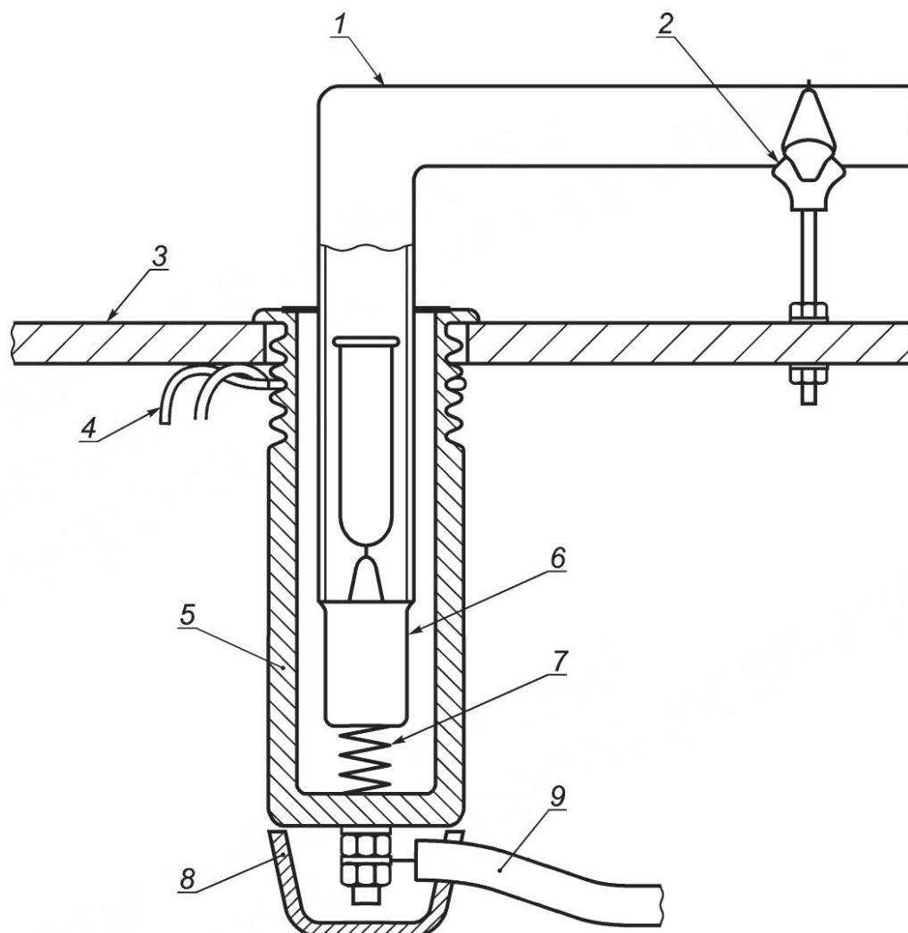
1 — газоразрядная лампа; 2 — опора для газоразрядной лампы в соответствии с требованиями 14.7.7; 3 — наружная поверхность ограждающей панели; 4 — зажим-фиксатор проводки; 5 — корпус электрода; 6 — электрод с металлической крышкой клемм; 7 — контактная пружина из фосфористой бронзы; 8 — изоляционная крышка; 9 — высоковольтный кабель
