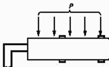
Рисунок 1 — Пример испытания светильника на ветровую нагрузку
