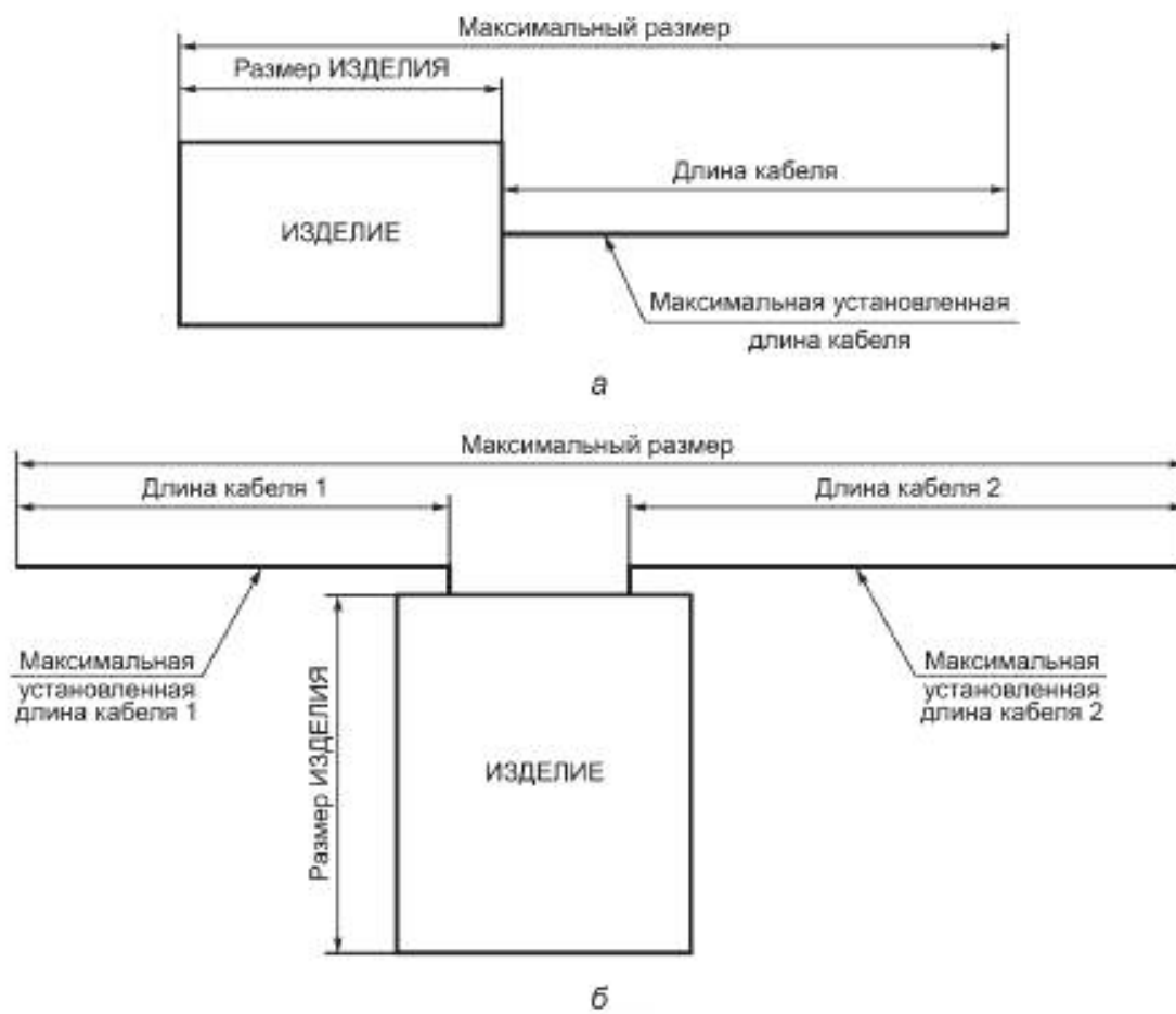
Рисунок А.2 — Примеры определения максимальных размеров МЕ ИЗДЕЛИЙ [см. 6.2.6.1 в) и ф)]: а — с одним кабелем; б — с двумя кабелями
