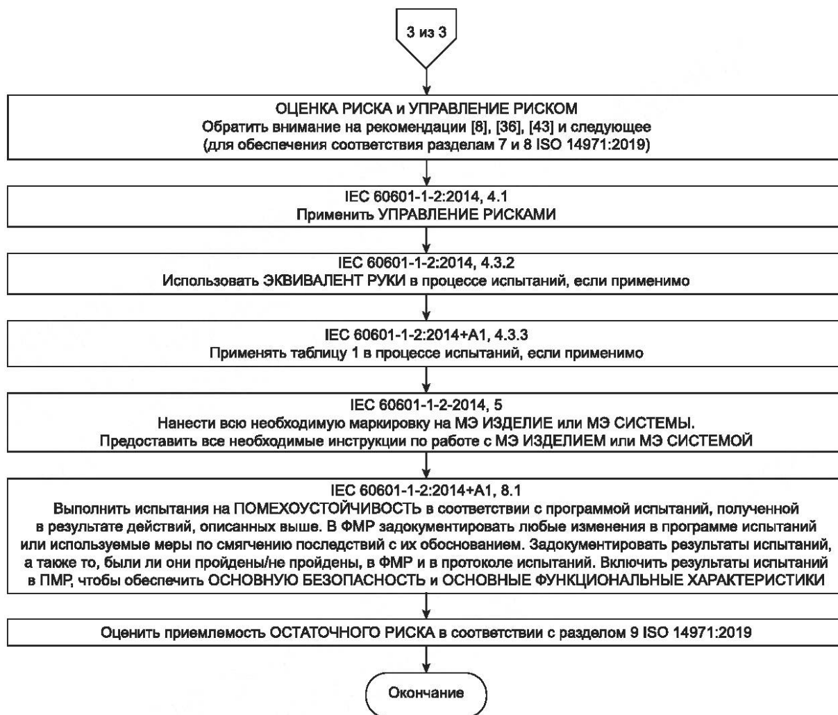
Рисунок F.3 — Процесс менеджмента риска в IEC 60601-1-2 (3 из 3)
