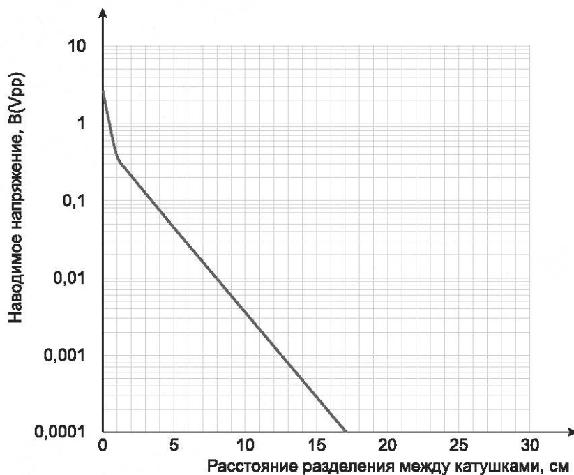
Рисунок А.6 — Напряжение, наводимое в одновитковой катушке радиусом 2 см от аналогичной катушки, работающей на частоте 13,56 МГц со среднеквадратическим значением напряженности магнитного поля 7,5 А/м
