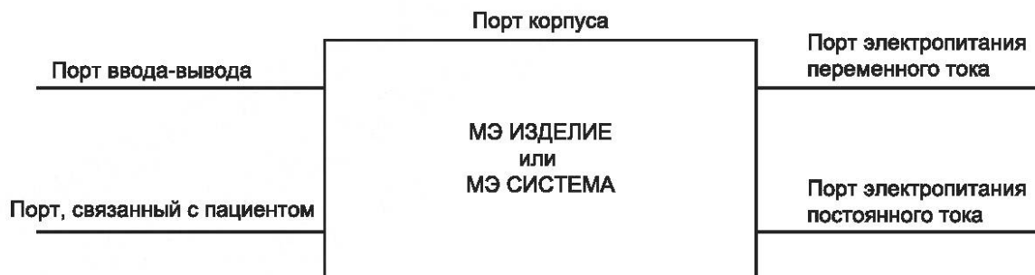
Рисунок 2 — Порты МЭ ИЗДЕЛИЙ и МЭ СИСТЕМ
