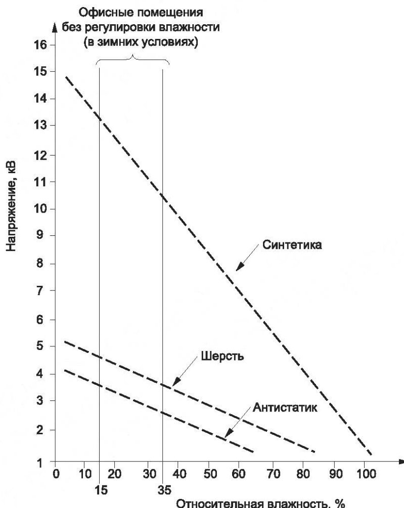
Рисунок А.2 — Максимальные значения напряжения, до которого могут быть заряжены операторы при контакте с материалами, приведенными в А.2 IEC 61000-4-2
