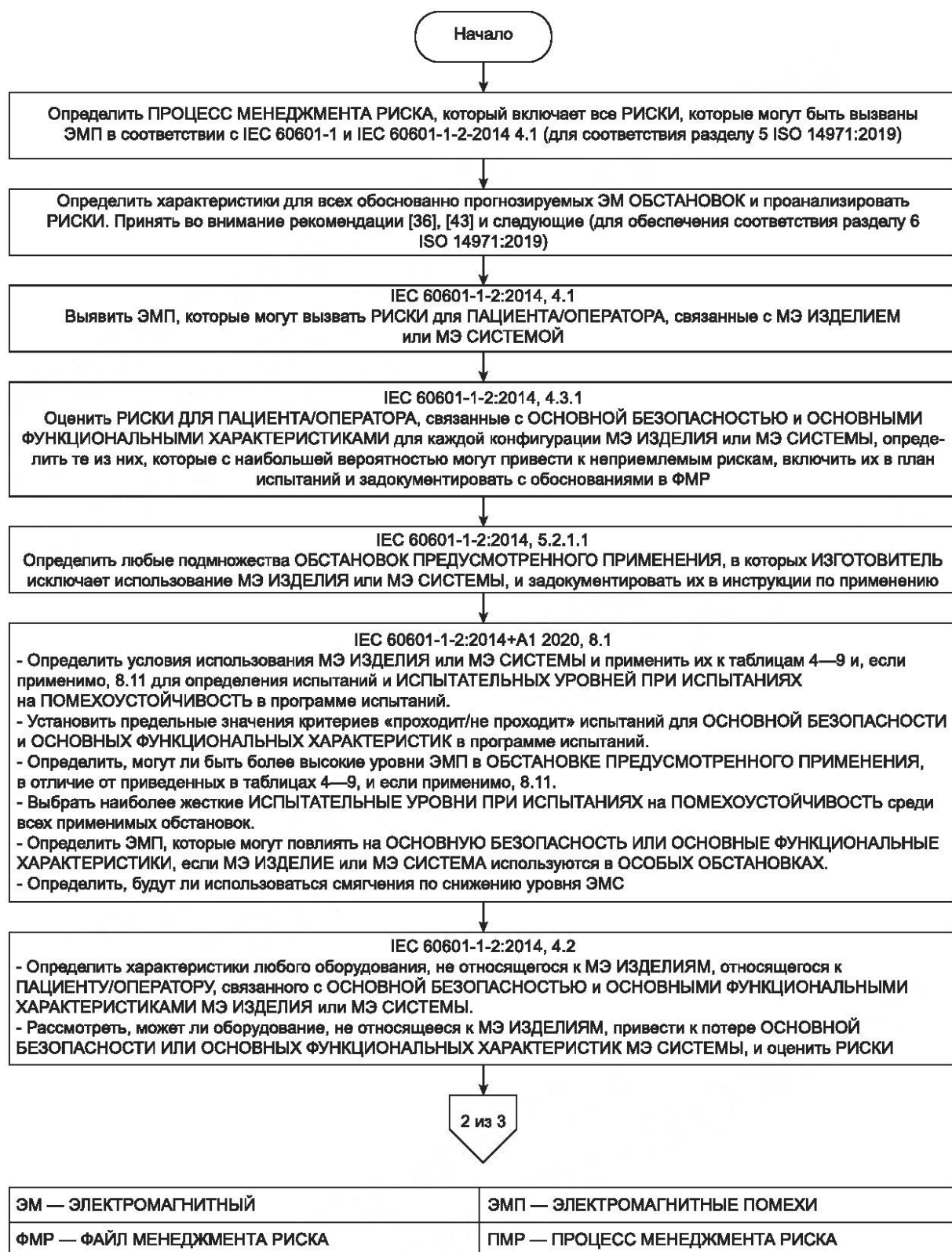
Рисунок F.1 — Процесс менеджмента риска в IEC 60601-1-2 (1 из 3)
