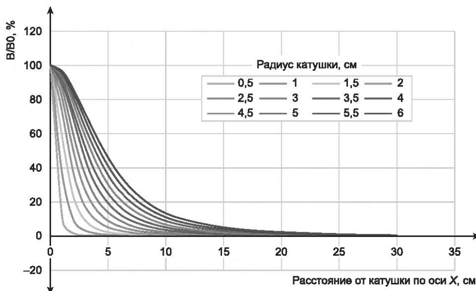
Рисунок А.4 — Характеристики затухания магнитного поля вдоль оси X для тонкой плоской катушки с различными радиусами
