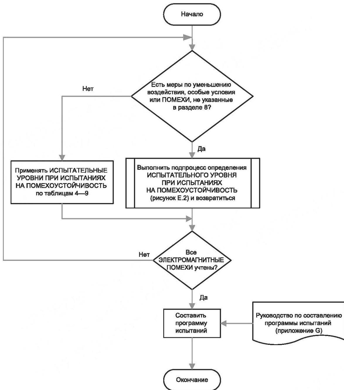
Рисунок Е.1 — Процесс разработки программы испытаний, если указаны ОСОБЫЕ ОБСТАНОВКИ
