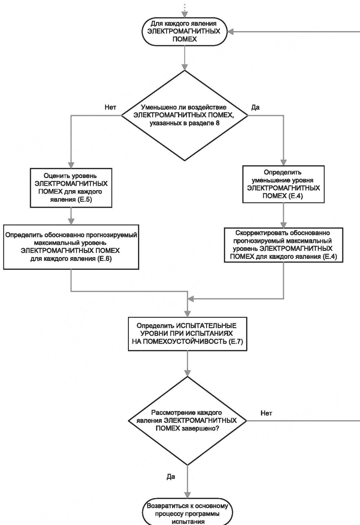
Рисунок E.2 — Подпроцесс определения ИСПЫТАТЕЛЬНЫХ УРОВНЕЙ ПРИ ИСПЫТАНИЯХ НА ПОМЕХОУСТОЙЧИВОСТЬ для ОСОБЫХ ОБСТАНОВКИ
