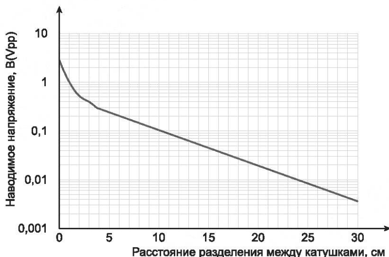
Рисунок А.5 — Напряжение, наводимое в одновитковой катушке радиусом 0,06 м от аналогичной катушки, работающей на частоте 134,2 кГц со среднеквадратическим значением напряженности магнитного поля 82,65 А/м
