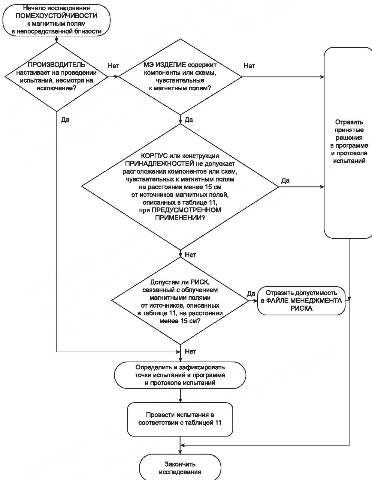
Рисунок А.3 — Пошаговое исследование ПОМЕХОУСТОЙЧИВОСТИ к магнитным полям в непосредственной близости
