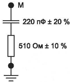
Рисунок 1 — RC-цепь эквивалента руки
