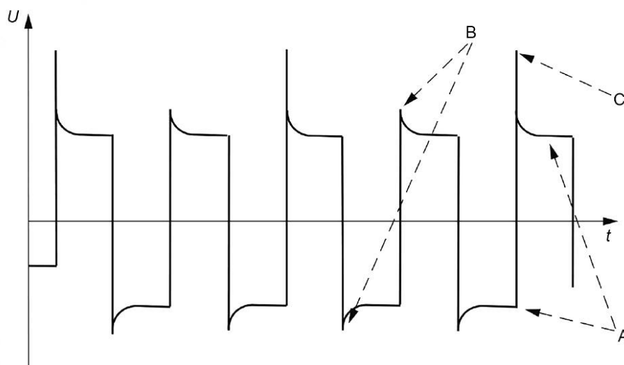
А — установившееся значение напряжения; В — установившееся пиковое напряжение; С — повторяющееся пиковое напряжение
