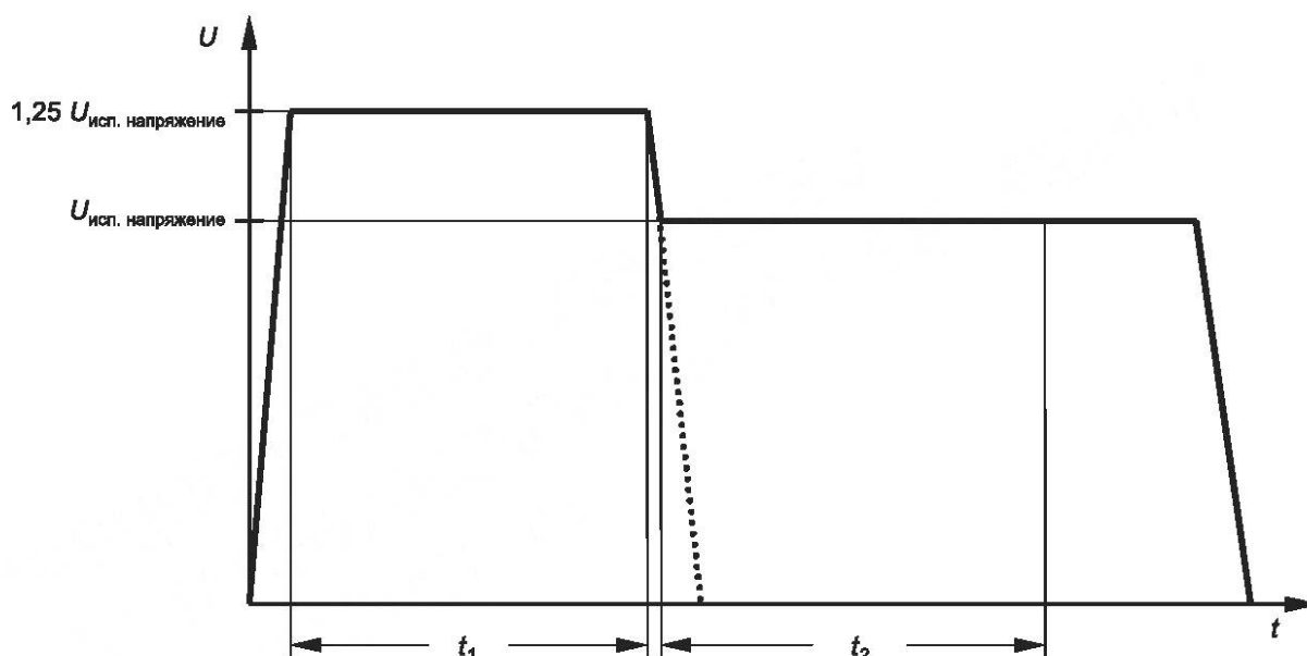
Рисунок 3 — Испытательные напряжения
