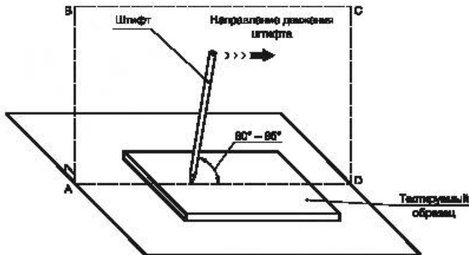
Рисунок 1 — Испытания на устойчивость к царапинам
