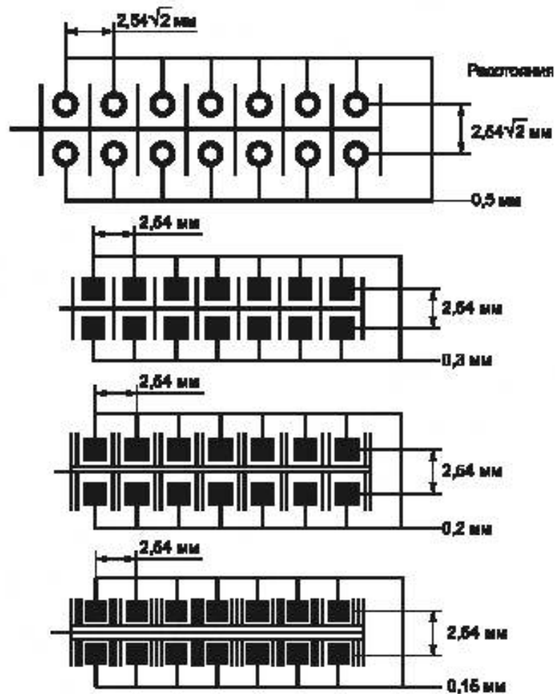
Рисунок С.2 — Конфигурация контактов и смежных с ними проводников
