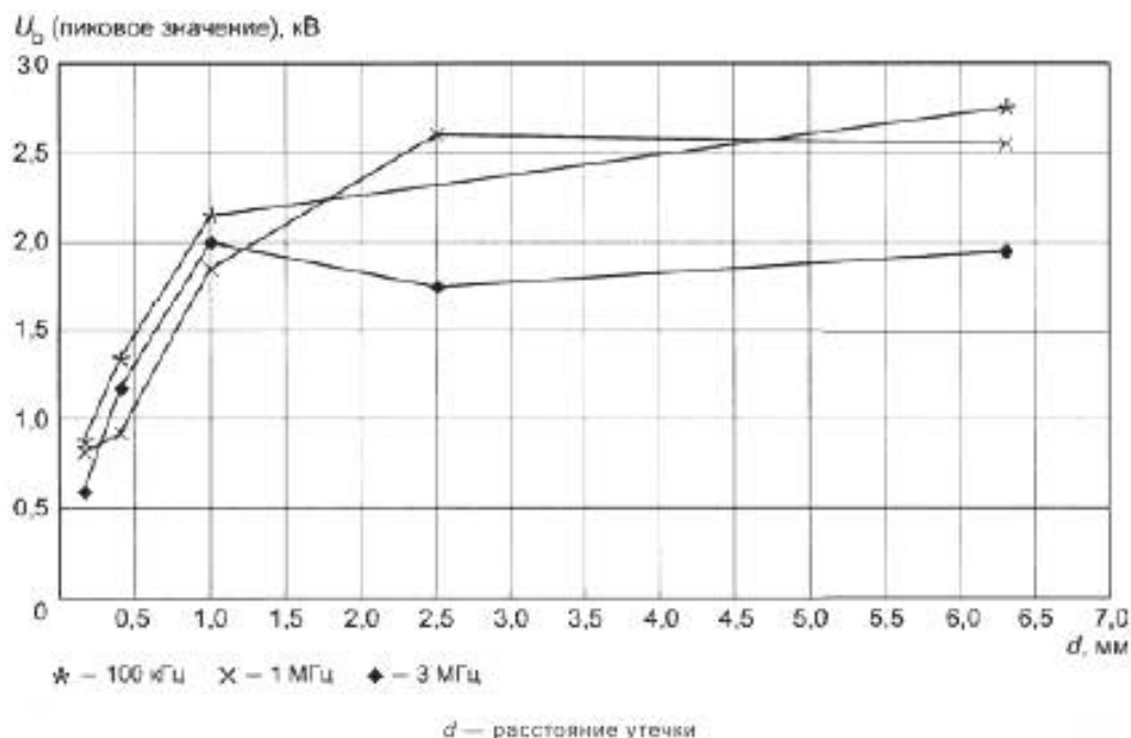
Рисунок В.3 — Результаты испытания напряжения пробоя U_b при расстояниях утечки не более 6,3 мм
