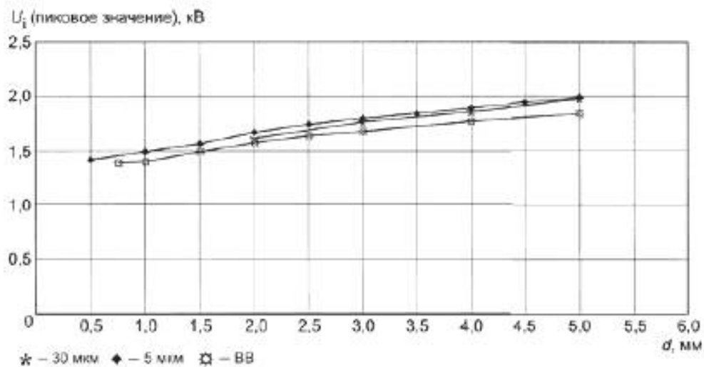
Рисунок А.4 — Начальное напряжение ЧП в воздухе при атмосферном давлении для частоты 100 кГц, точечные электроды с различными радиусами точки
