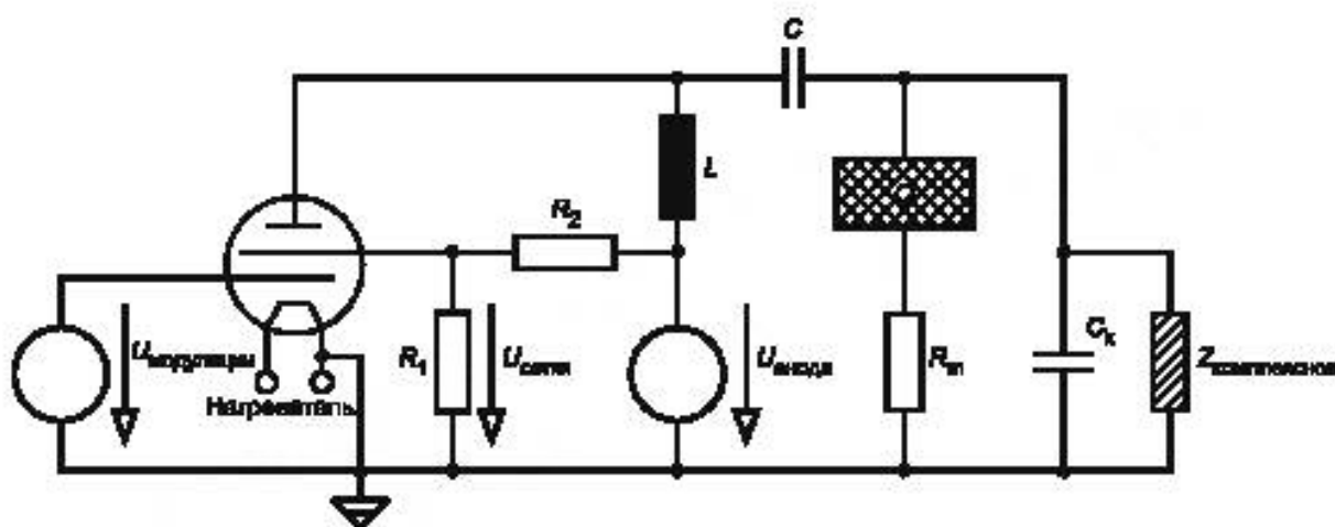
Рисунок D.2 — Высокочастотный генератор большой мощности [5] и [6]
