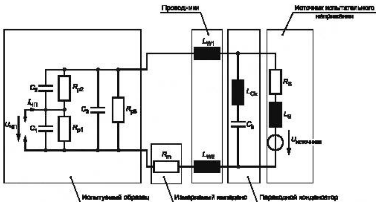
Рисунок D.6 — Эквивалентная цепь испытания тока ЧП с общими элементами
