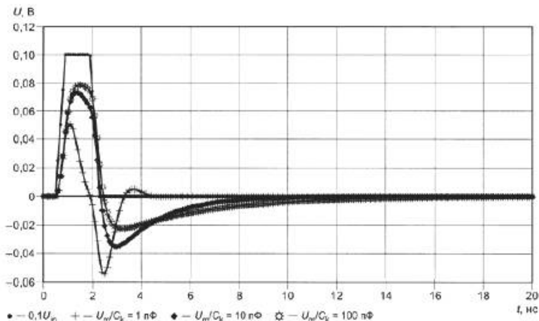
Рисунок D.8 — Входной сигнал U_{\text{в}} и измеряемый сигнал U_{\text{из}} , зависящие от емкости конденсатора связи C_k (емкость испытуемого образца C_3 = 10 пФ) [5]
