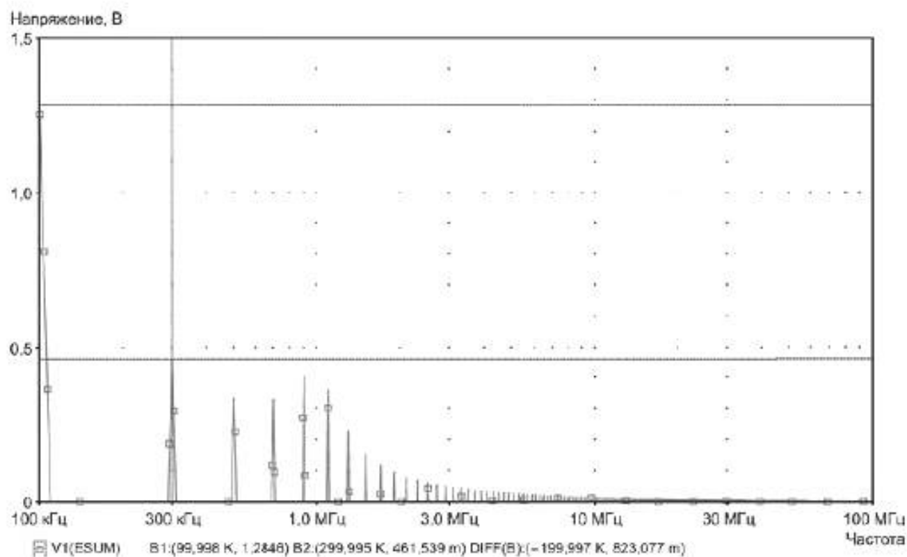
Рисунок Е.6 — Периодические импульсы напряжения, прямоугольная форма волны с всплесками (частота 1 МГц), анализ спектра частот
