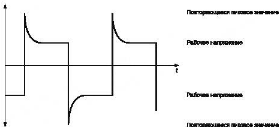
Рисунок 4 — Периодическое импульсное напряжения (см. IEC 60664-1)
