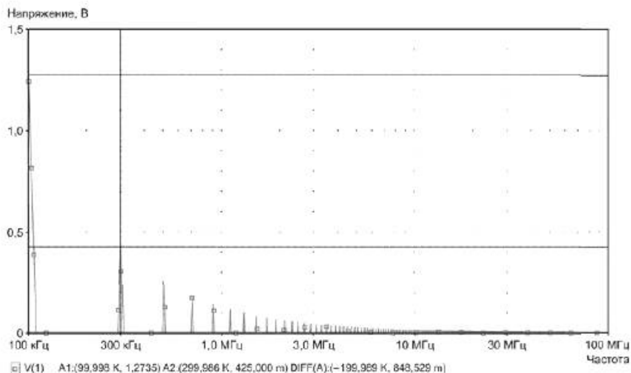
Рисунок Е.2 — Периодические импульсы напряжения, прямоугольная форма волны, анализ спектра частот
