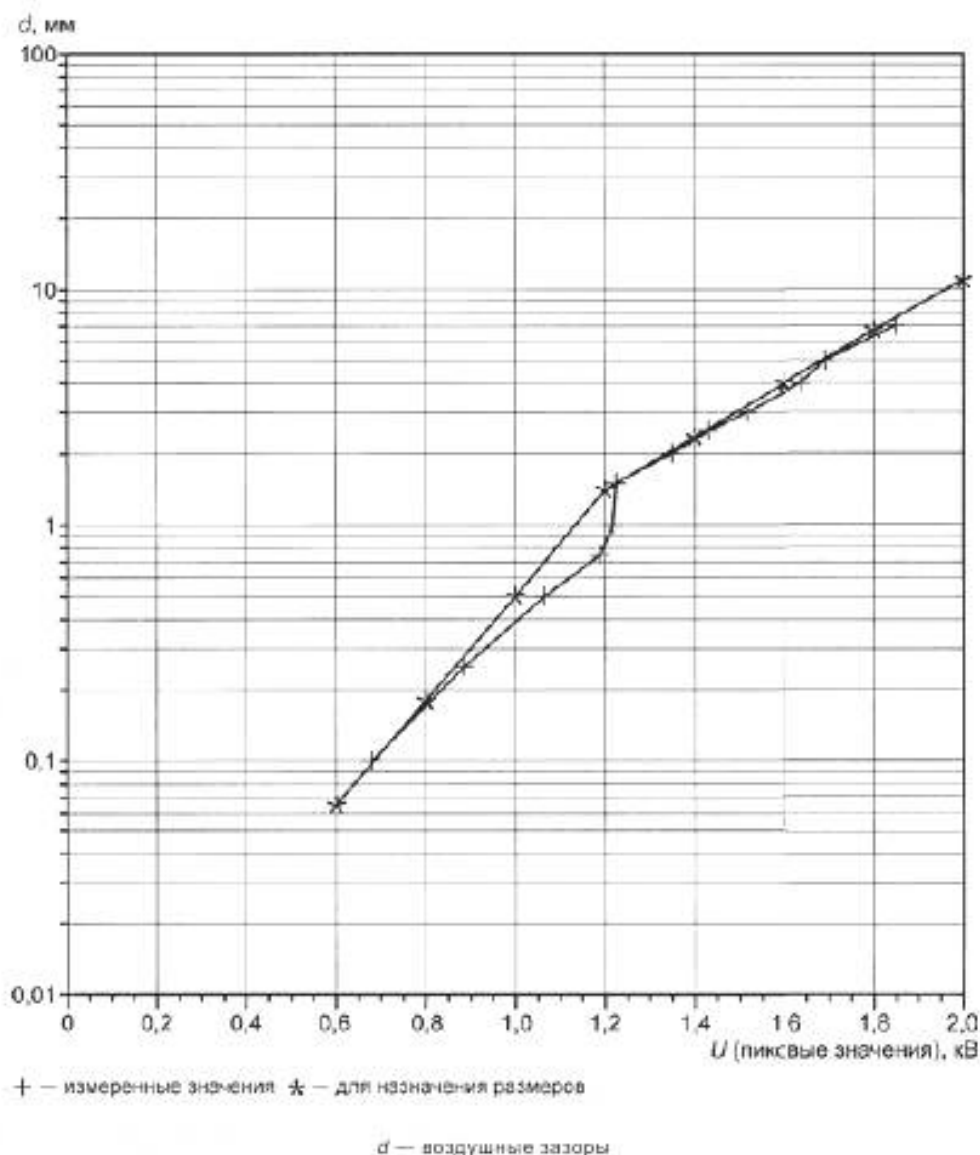
Рисунок 1 — Размеры воздушных промежутков в неоднородном поле в воздушной среде при атмосферном давлении (радиусы точек электродов в плане — 5 мкм) для исключения случаев ЧП или пробоев (воздушные зазоры менее 1 мм)
