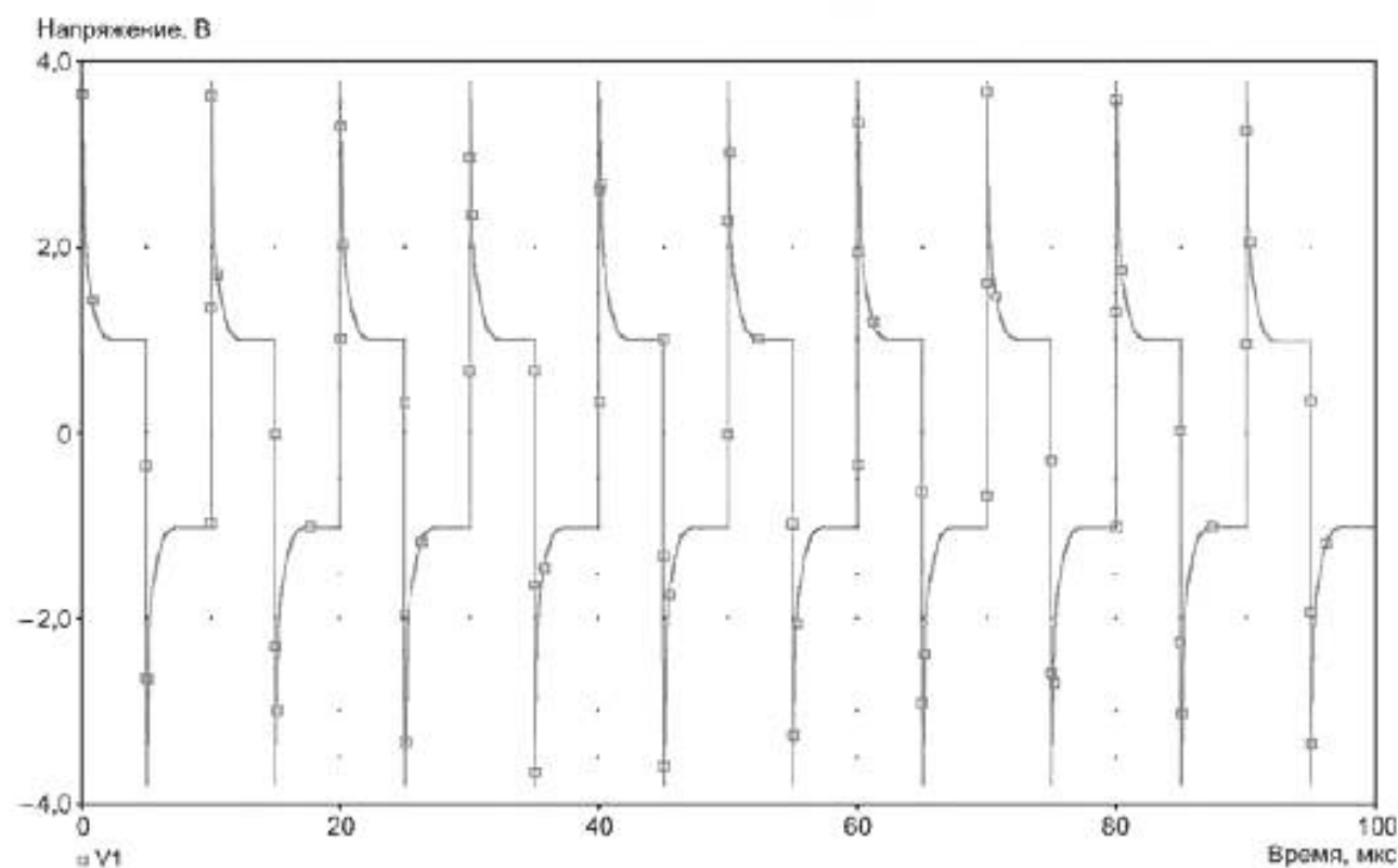
Рисунок Е.7 — Периодические импульсы напряжения, прямоугольная форма волны со значительными всплесками
