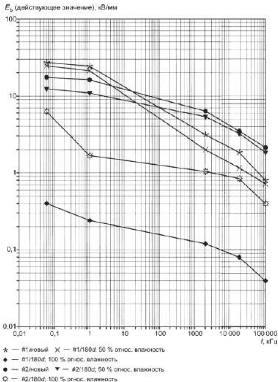
Рисунок С.4 — Высокочастотный пробой твердой изоляции, влияние влажности; условия при 50 °C: #1: наполненный слюдой фенол, d = 0,75 мм; #2: ламинат из кремнивого стекла, d = 0,75 мм [19]
