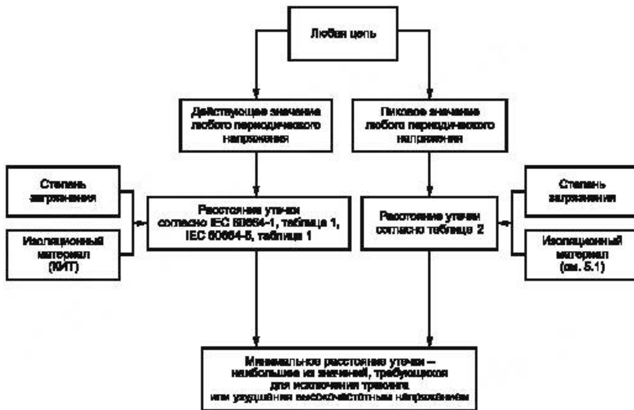
Рисунок F.2 — Диаграмма определения расстояний утечки
