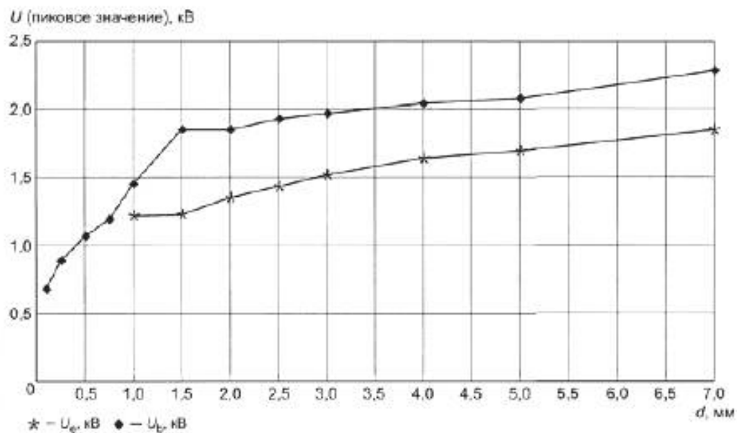
Рисунок А.6 — Напряжения затухания ЧП и напряжения пробоя в воздухе при атмосферном давлении для частоты 1 МГц, точечные электроды с ВВ-иглами [6]
