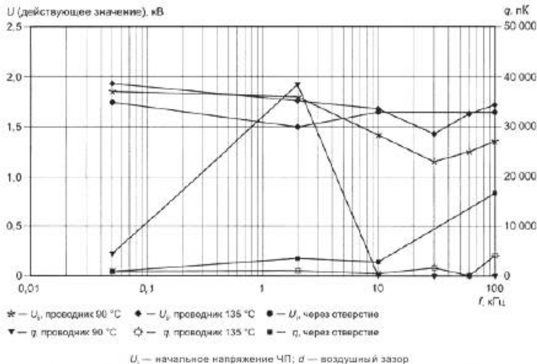
Рисунок D.11 — Испытание ЧП покрытых печатных плат; U_0 , d = 0,2 мм [30]
