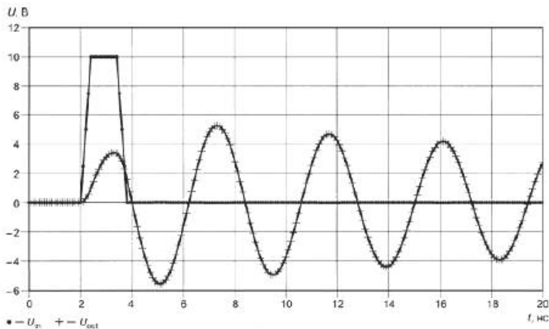
а — Импульс ЧП источника напряжения
