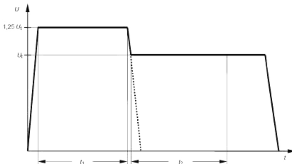
Рисунок 1 – Испытательное напряжение
