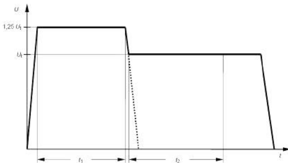
Рисунок 1 – Испытательное напряжение
