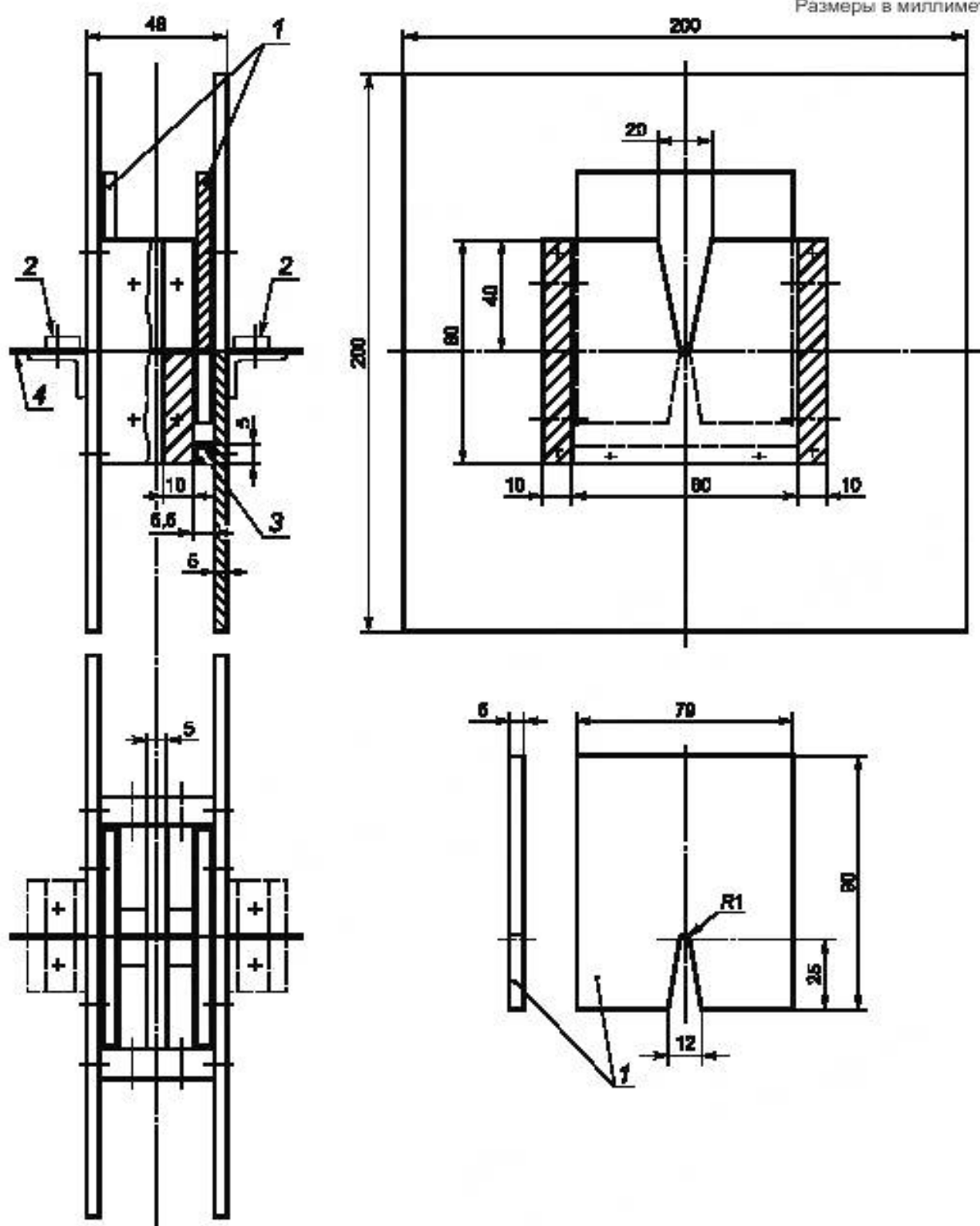
Рисунок 105 — Испытательная установка для проверки минимальных значений \rho_t и I_p , выдерживаемых разъединителем
