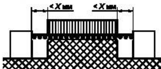
Рисунок АА.4 — Ребро
