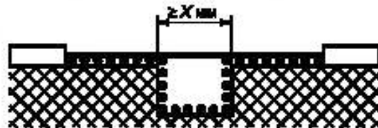
Рисунок АА.1 — Узкий желобок
