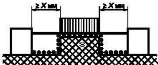
Рисунок АА.5 — Нескрепленный стык с узким желобком
