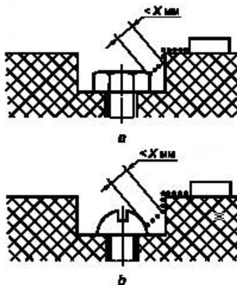
Рисунок АА.9 — Узкий паз
