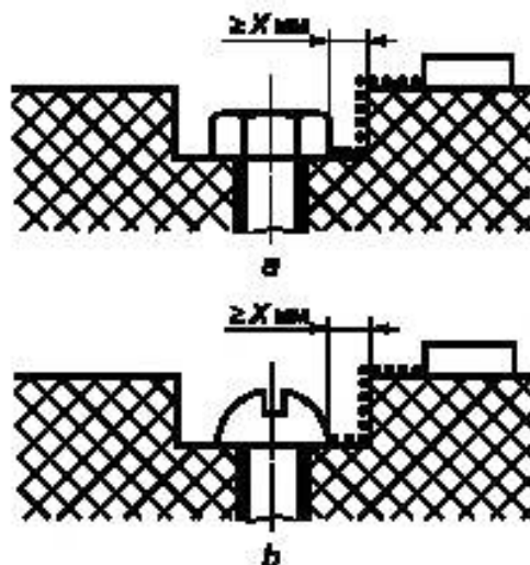
Рисунок АА.10 — Широкий паз
