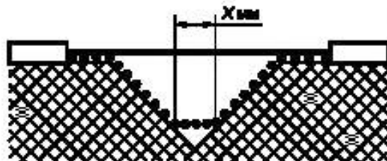
Рисунок АА.2 — Широкий желобок
