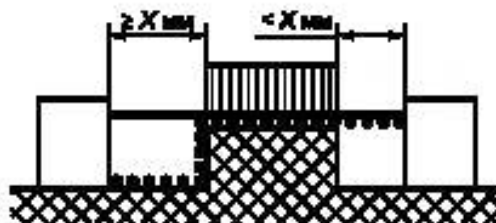
Рисунок АА.6 — Нескрепленный стык с широким желобком
