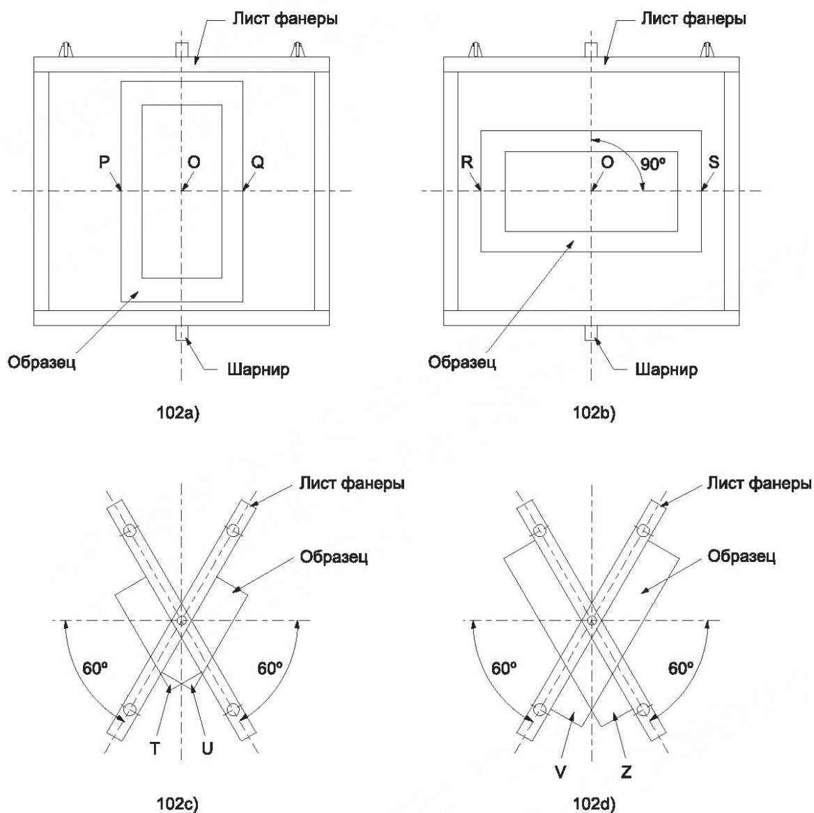
Рисунок 102 — Схемы нанесения ударов, лист 1
