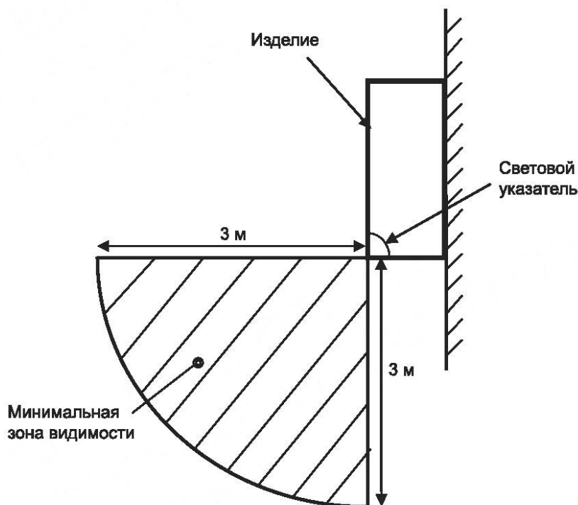
Рисунок 101 — Минимальная зона видимости
