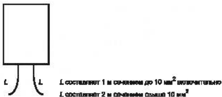
Рисунок 101 — Одиночное оконечное устройство
