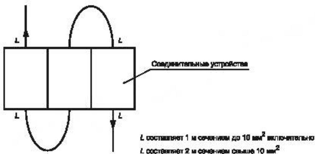
Рисунок 102 — Многопозиционное оконечное устройство
