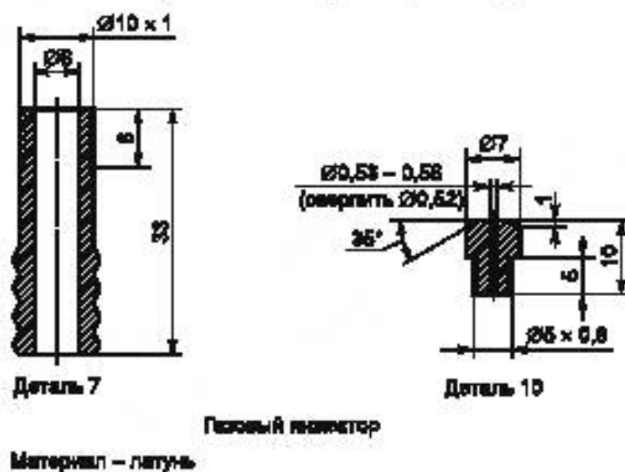
Рисунок А.4 — Детали горелки (3)
