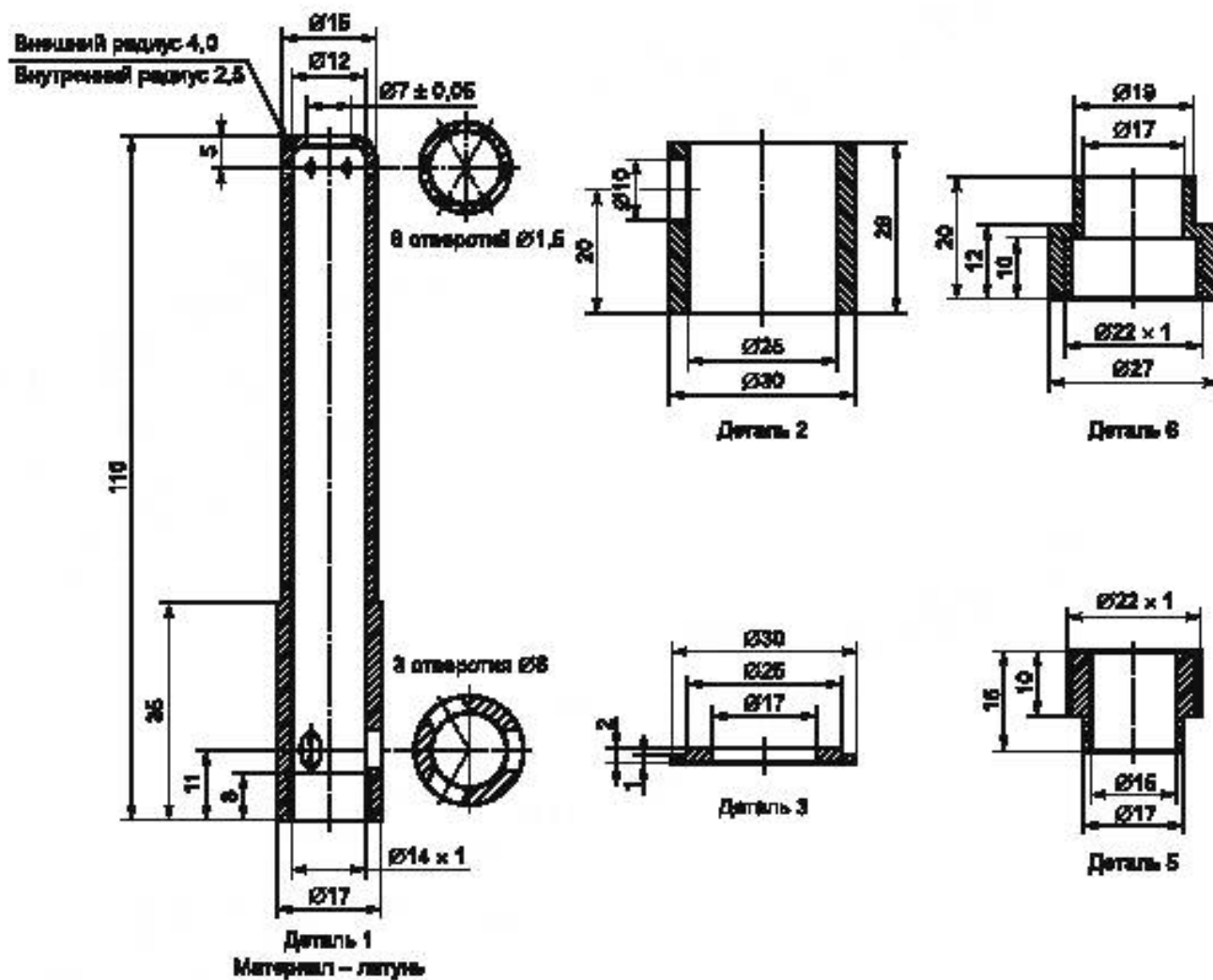
Рисунок А.2 — Детали горелки (1)
