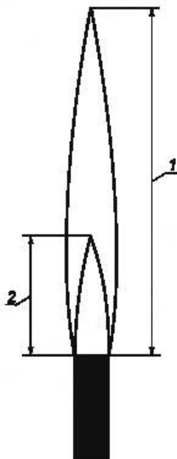
Рисунок 1 — Размеры пламени
