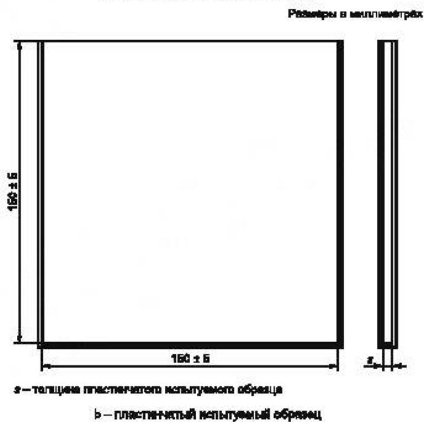
Рисунок 4 — Испытуемые образцы
