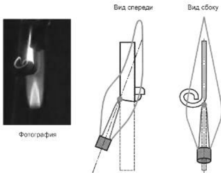
Рисунок A.3 — Точка приложения пламени для закрученного образца
