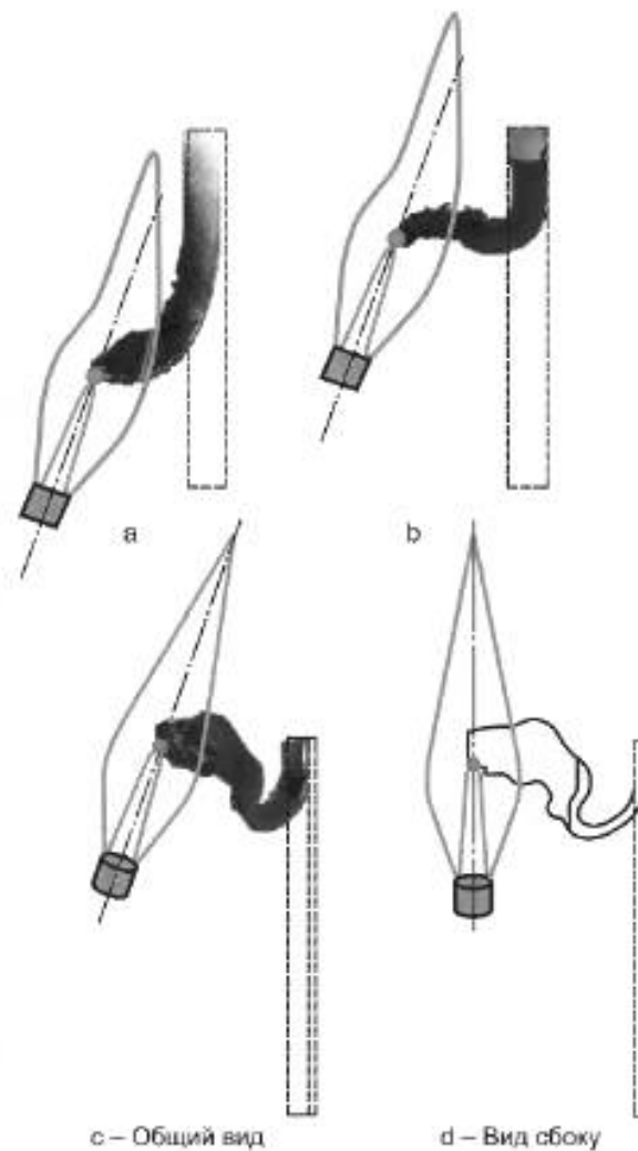
Рисунок A.3 — Точка приложения пламени для закрученного образца
