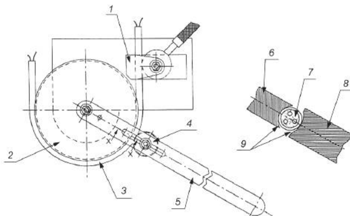
1 — зажим; 2 — оправка; 3 — кабель; 4 — ролик; 5 — рычаг для изгиба; 6 — оправка; 7 — кабель; 8 — ролик; 9 — радиус канавок; x — x фрагмент в увеличенном масштабе
