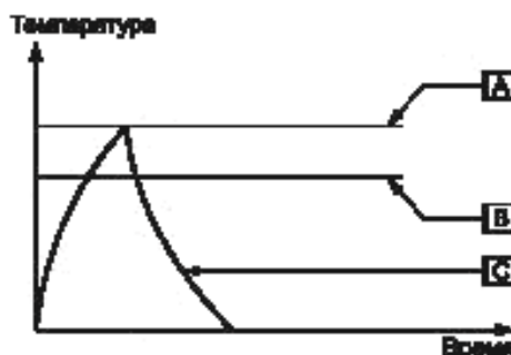
Рисунок EE.3 — Термоограничитель без самовозрата
