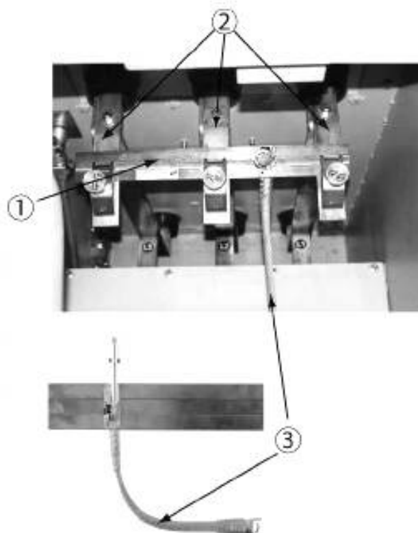
1 — короткозамыкающая шина; 2 — проводники; 3 — кабель заземления
