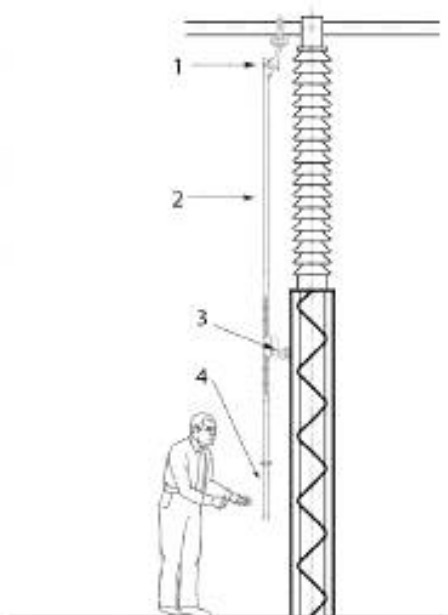
1 — копьевой контакт на проводнике; 2 — копьё; 3 — неподвижная точка заземления; 4 — изолированная ручка
