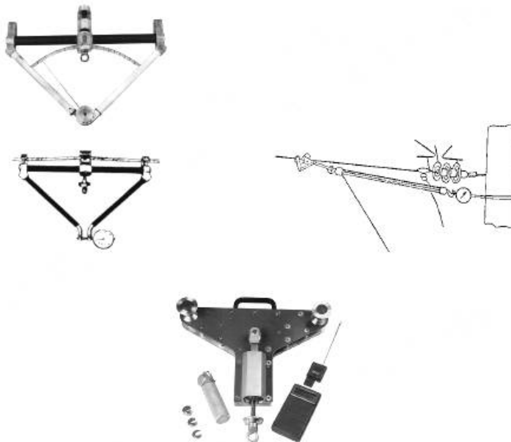
Различные конструкции динамометров
