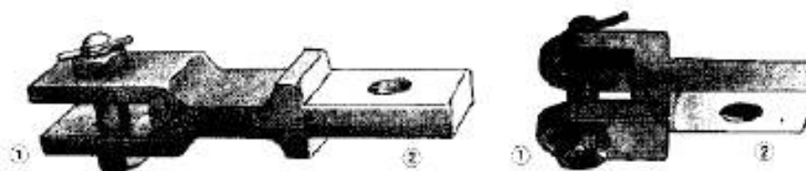
1 — вилка; 2 — однолапчатая проушина
