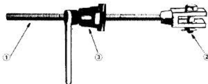
1 — винт; 2 — вилка; 3 — трещотка
