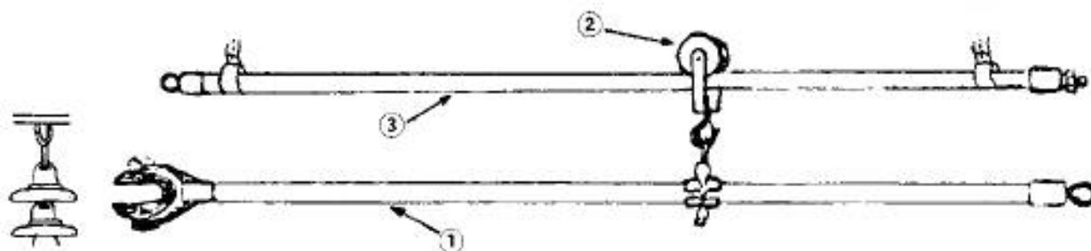
1 — штанга поддержки изолятора; 2 — контактный ролик; 3 — штанга каретки
