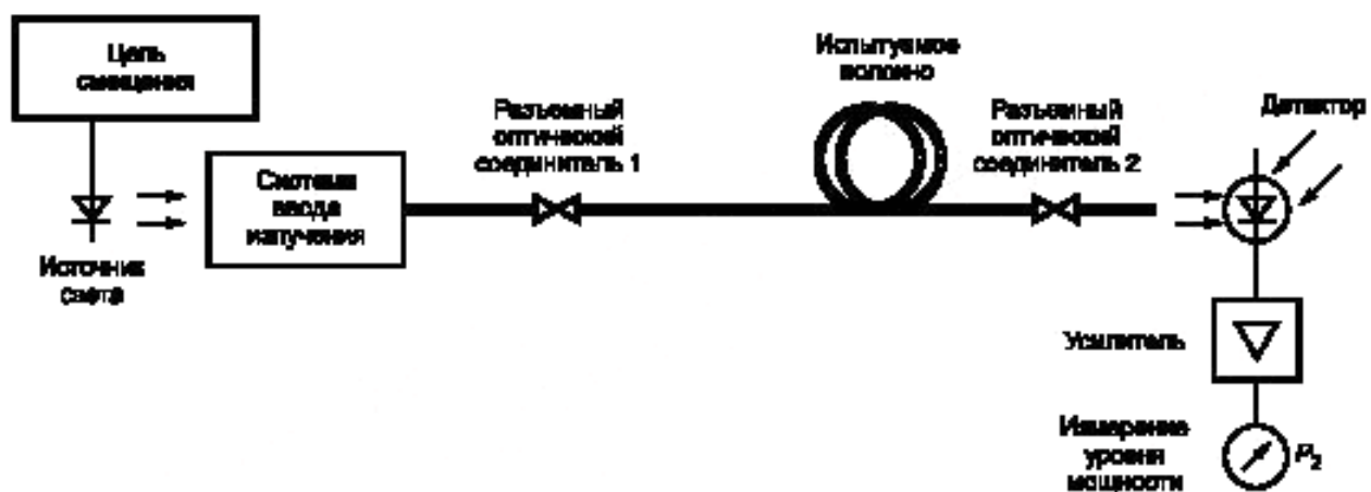
Рисунок В.2 — Измерение вносимых потерь
