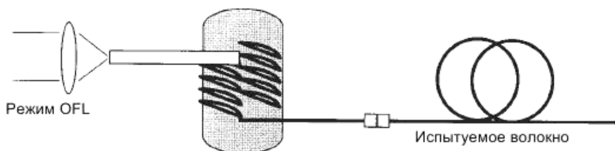
Рисунок 1 – Модовый фильтр, намотанный на оправку
