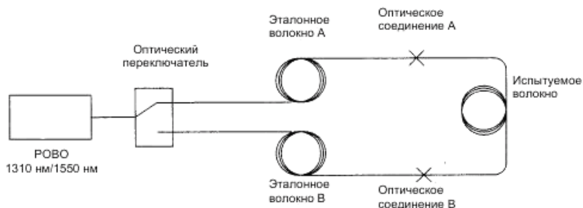
Рисунок D.1 – Расположение оптического переключателя
