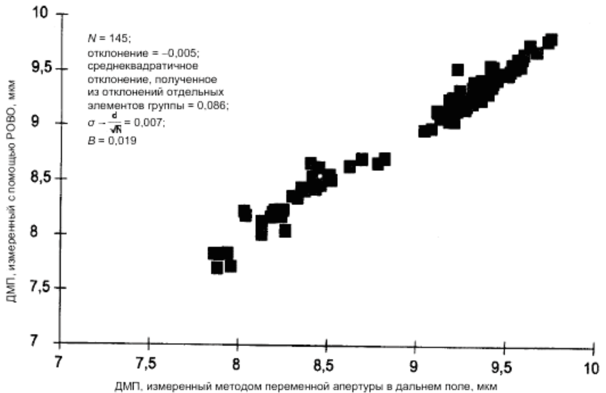
Рисунок D.4 – Пример проверки достоверности результатов измерений. Сравнение методов
