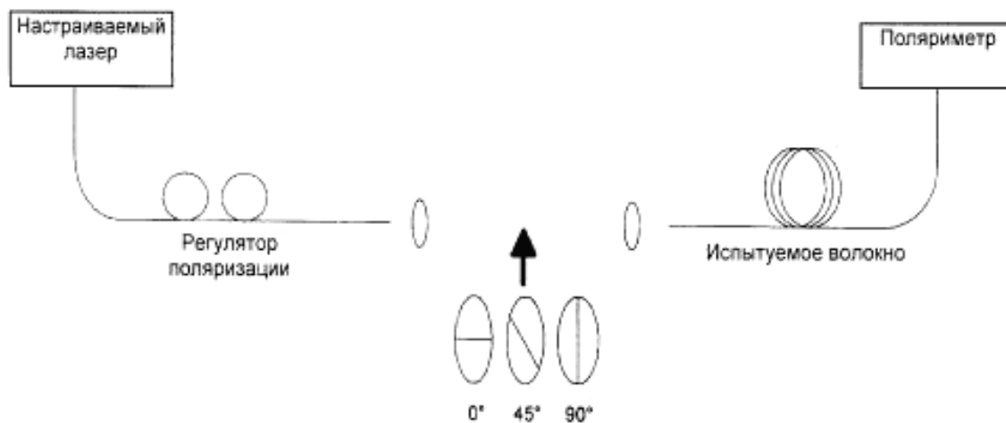
В.1а – узкополосный источник (JME)
