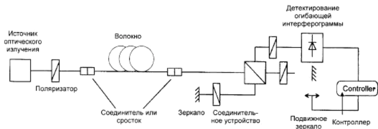
С.2а – интерферометр Михельсона
