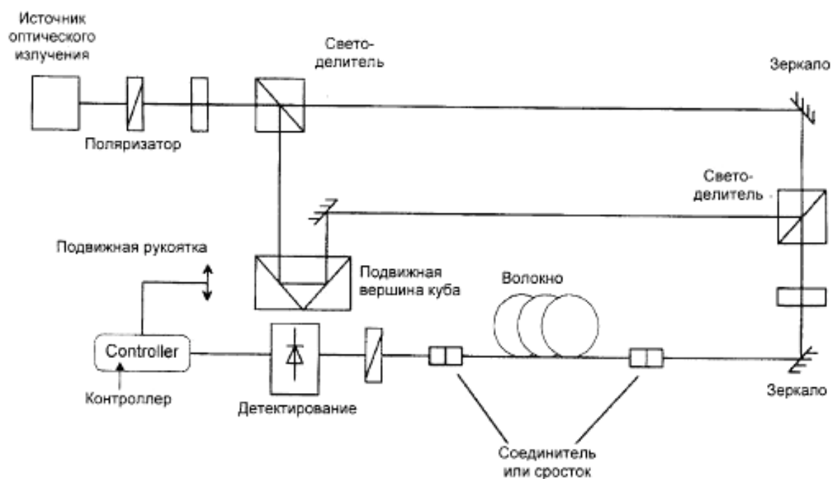
С.2b – интерферометр Маха-Зандера
