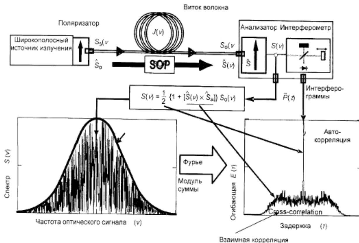
Рисунок С.1 – Блок-схема для метода С (типовая реализация)
