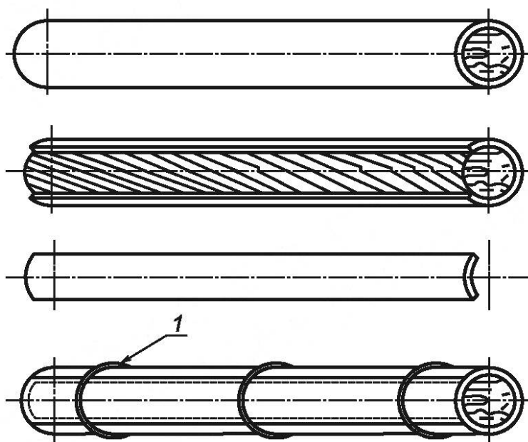
Рисунок В.1 — Специально подготовленные испытываемые образцы
