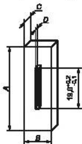
Рисунок 7 — Образец с надрезом
