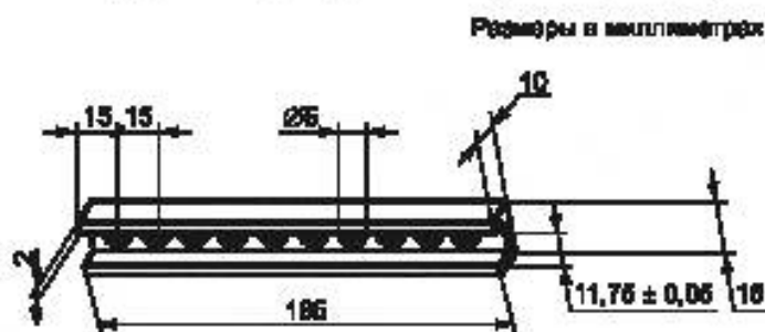
Рисунок 5 — Латунный профильный держатель образцов
