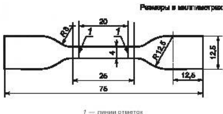
Рисунок А.1 — Образец в виде двусторонней лопатки
