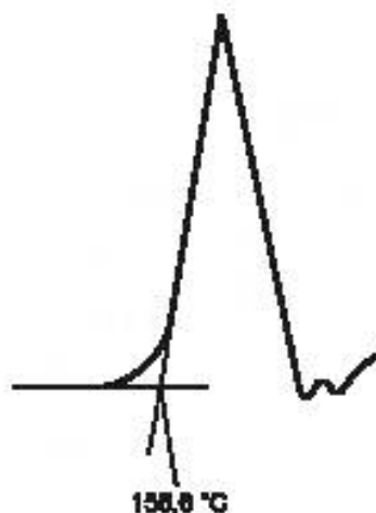
Рисунок А.1 — Эндотерма плавления индия
