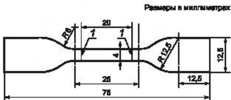
Рисунок 1 — Образец в форме двусторонней лопатки
