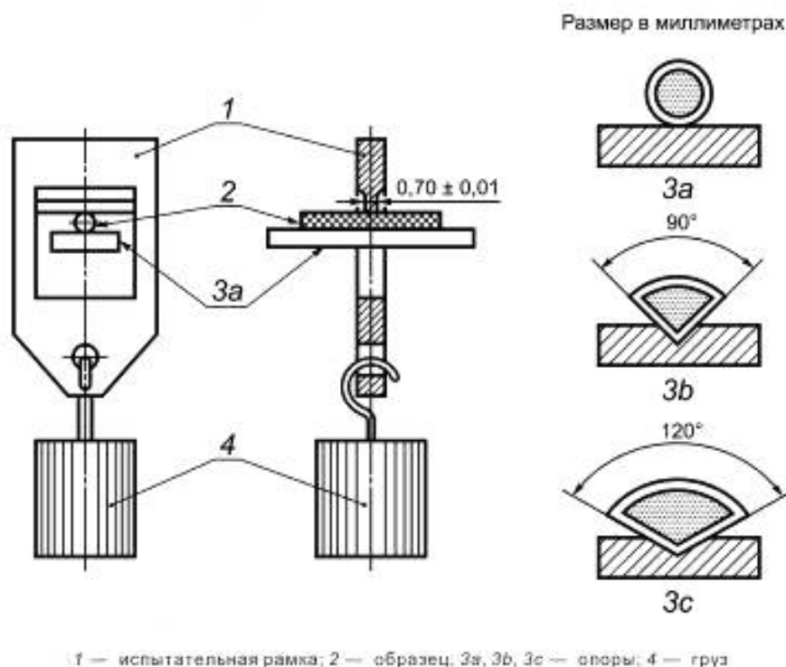
Рисунок 1 — Устройство для продавливания образца
