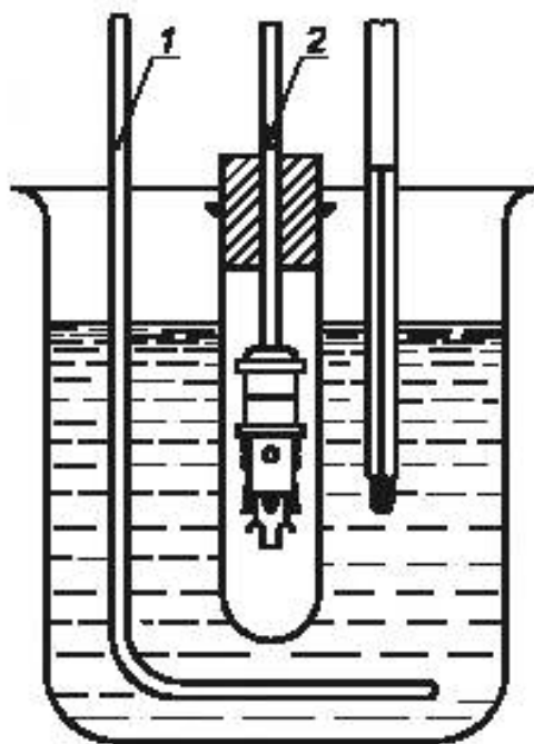
1 — мешалка; 2 — линия погружения
