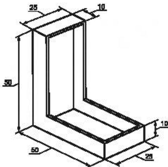
Рисунок 1 — Угловой бокс с двумя прямоугольными ящиками
