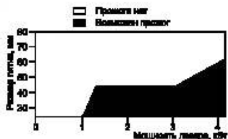
Рисунок F.20 — Стойкость к разрушению листа алюминия толщиной 2 мм от 100 с экспозиции расфокусированного пучка во время экспериментов с использованием непрерывного лазера на иттрий-алюминиевом гранате с неодимом
