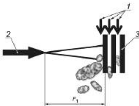
1 — Боковой поток воздуха, вентилирующий переднюю поверхность защиты и все ее внутренние пространства; 2 — пучок лазера; 3 — система защиты
