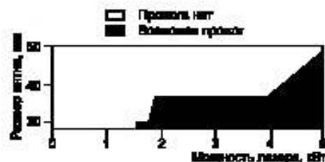
Рисунок F.7 — Стойкость к разрушению листа алюминия толщиной 2 мм от 10 с экспозиции расфокусированного пучка во время экспериментов с использованием непрерывного лазера на углекислом газе
