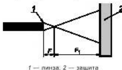
Рисунок D.1 — Упрощенная схема испытательной установки
