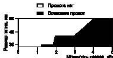
Рисунок F.9 — Стойкость к разрушению листа нержавеющей стали толщиной 1 мм от 10 с экспозиции расфокусированного пучка во время экспериментов с использованием непрерывного лазера на углекислом газе
