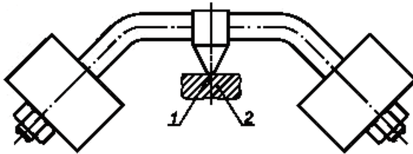
1 — сфера R = 2,5 мм; 2 — образец
