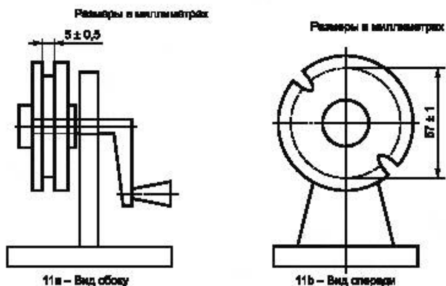
Рисунок 11 — Устройство для намотки
