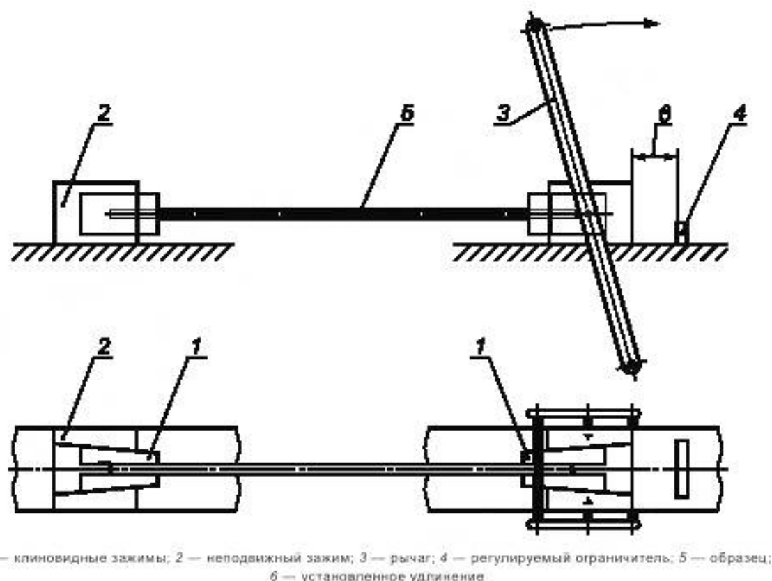
Рисунок 5 — Устройство для испытания рывком
