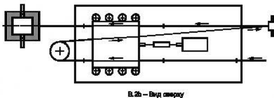
Рисунок В.2 — Испытательное устройство для определения динамического коэффициента трения
