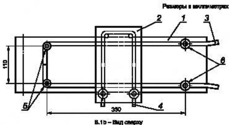
Рисунок В.1 — Испытательное устройство для определения статического коэффициента трения
