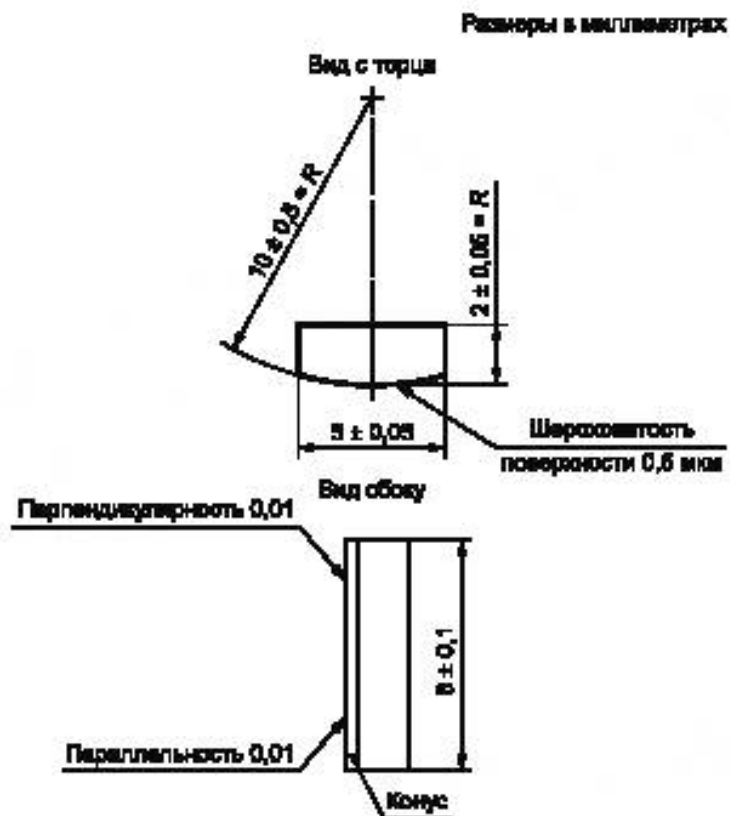
Рисунок В.4 — Материал — сапфир (синтетический)
