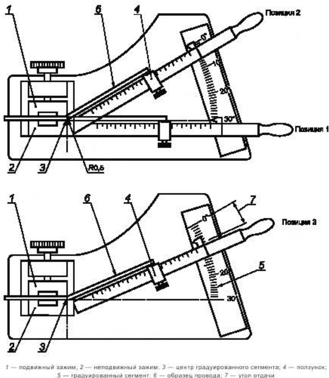
Рисунок 3 — Испытательное устройство для определения упругости
