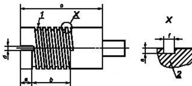
1 — канавка на 7 витков; 2 — часть X с увеличением
