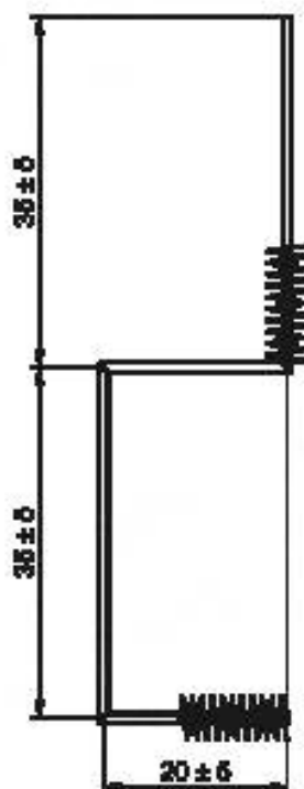
Рисунок 4 — Пример держателя для испытания на облуживание
