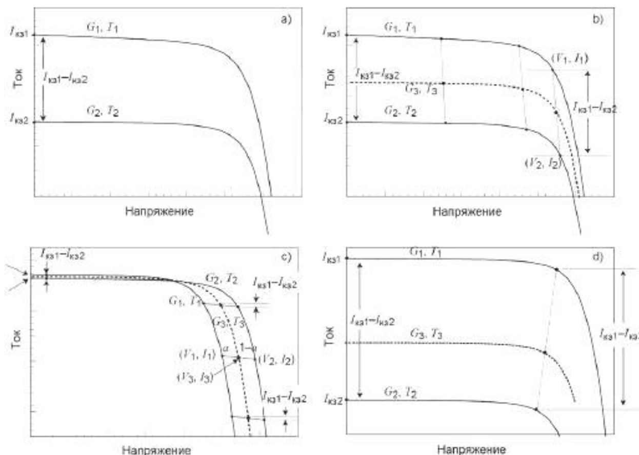
Рисунок 1 – Пример коррекции ВАХ с применением уравнений (6) и (7.) Рисунки (а) и (b) изображают коррекцию по энергетической освещенности, Рисунок (с) изображает коррекцию по температуре и Рисунок (d) – коррекцию одновременно по энергетической освещенности и температуре.
