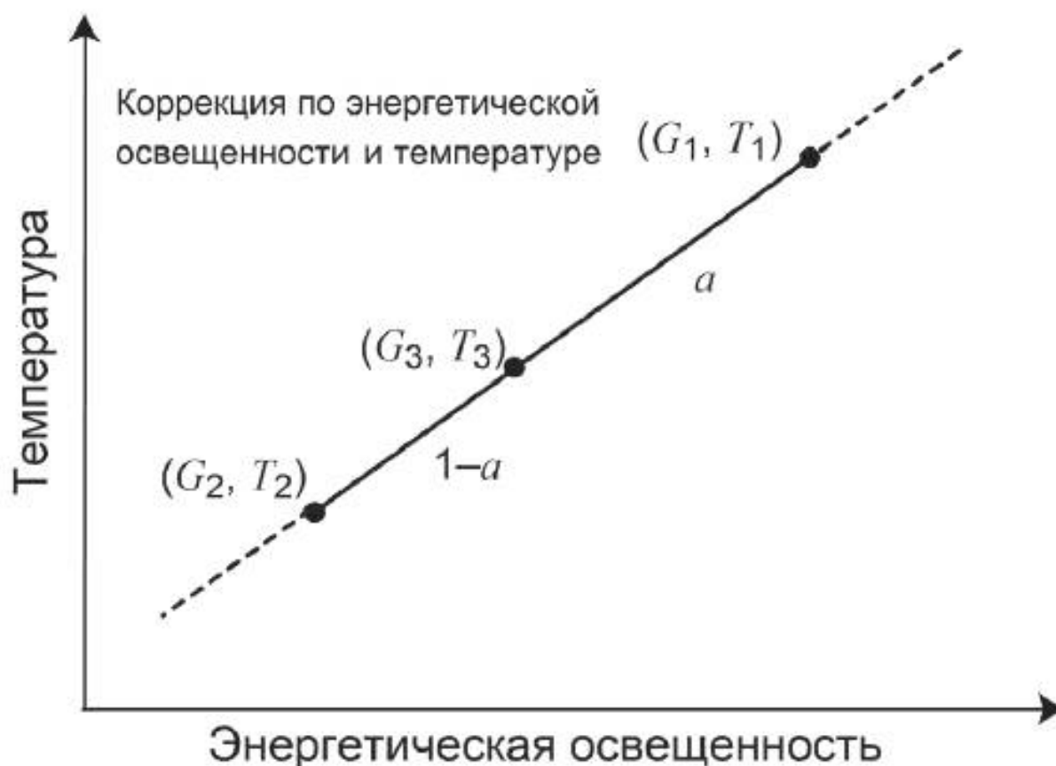
Рисунок 2 – Схематическая диаграмма соотношения значений G_3 и T_3 , которые могут быть выбраны с помощью уравнений (8) и (9) для фиксированных значений T_1 , G_1 , T_2 и G_2 при коррекции одновременно по энергетической освещенности и температуре. Непрерывная прямая и пунктирная прямая иллюстрируют диапазоны значений, в которых вычисляют G_3 и T_3 путем интерполяции и экстраполяции, соответственно.
