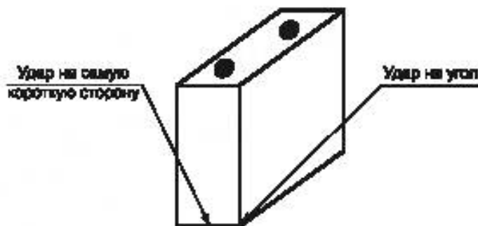
Рисунок 9 — Места на образце для удара
