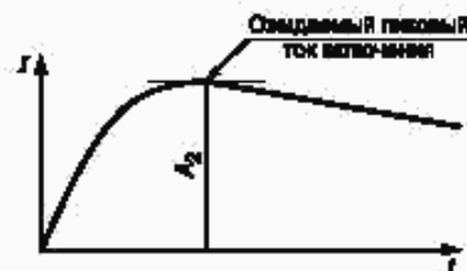
Рисунок 7b — Калибровка испытательной цепи для постоянного тока
