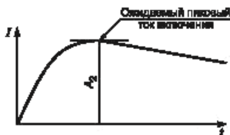
Рисунок 7b — Калибровка испытательной цепи для постоянного тока
