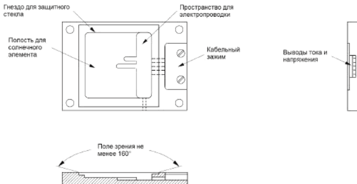
Рисунок 2 – Корпусирование одиночного солнечного элемента.
