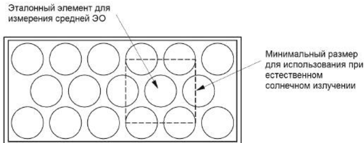
Рисунок 1 – Пример эталонного солнечного элемента в многоэлементном корпусе
