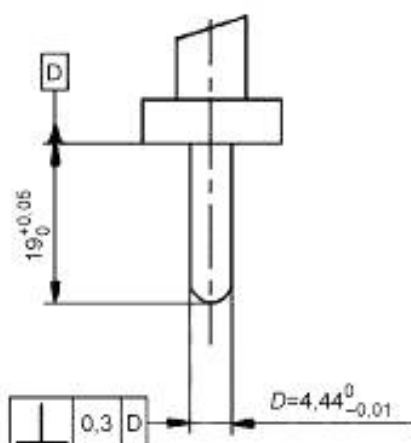
Рисунок 6 — Система вилок и штепсельных розеток на 16 А, 250 В переменного тока. Калибр для проверки минимального извлекающего усилия (IEC 60884-1, подраздел 22.2)
