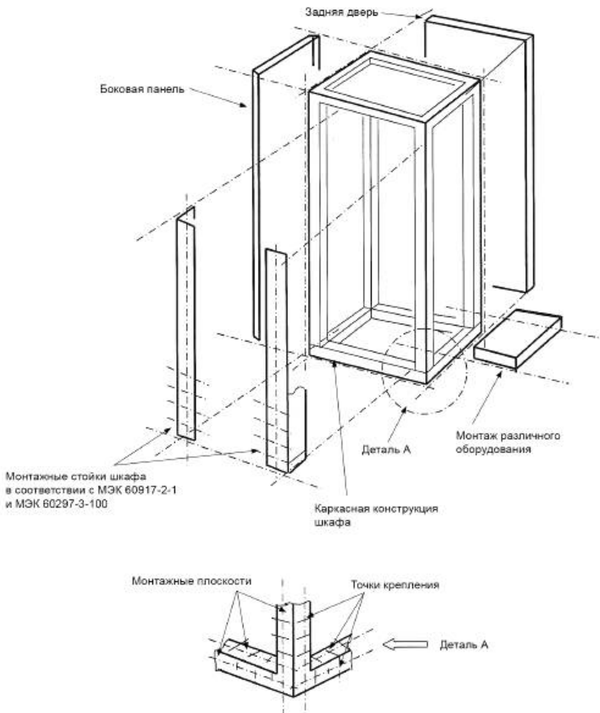
Рисунок 1 — Общая компоновка шкафа модульной базовой конструкции
