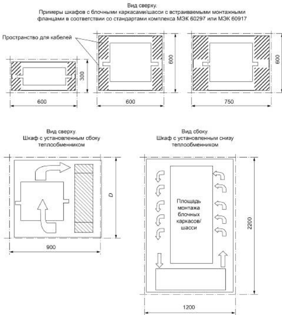
Рисунок А.2 — Примеры компоновки вспомогательного оборудования
