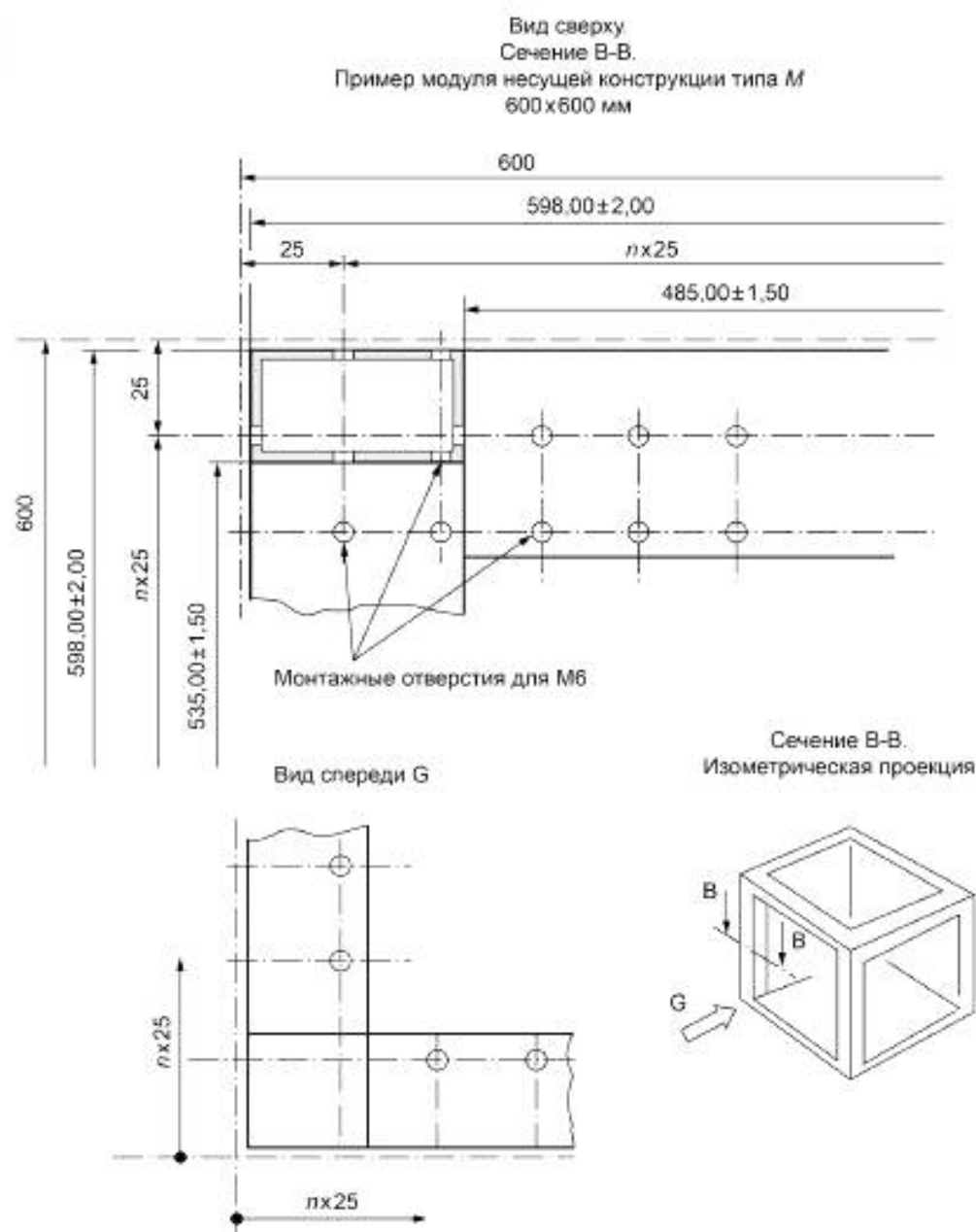
Рисунок 4 — Модуль несущей конструкции типа М 600 × 600 мм
