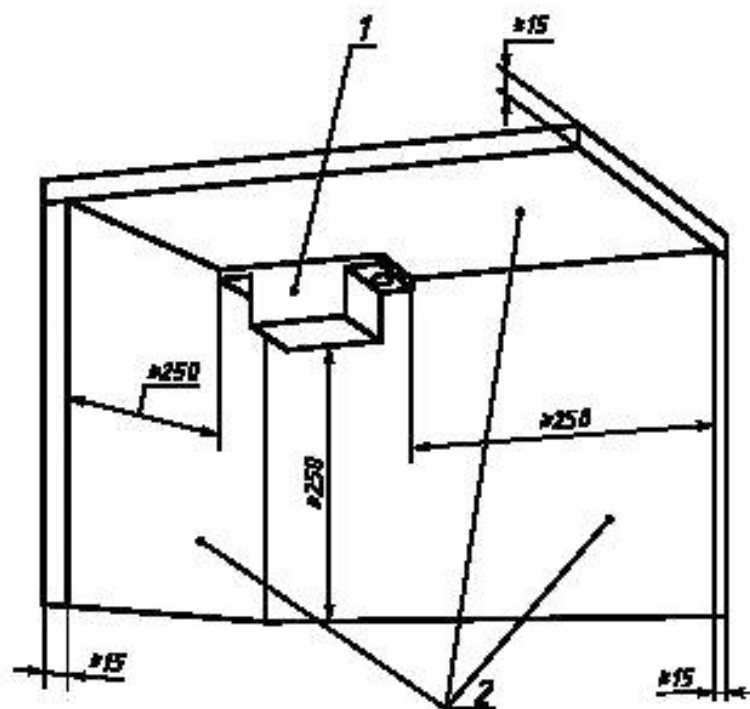
Рисунок 7 — Испытательный угол для тепловых испытаний ПРА
