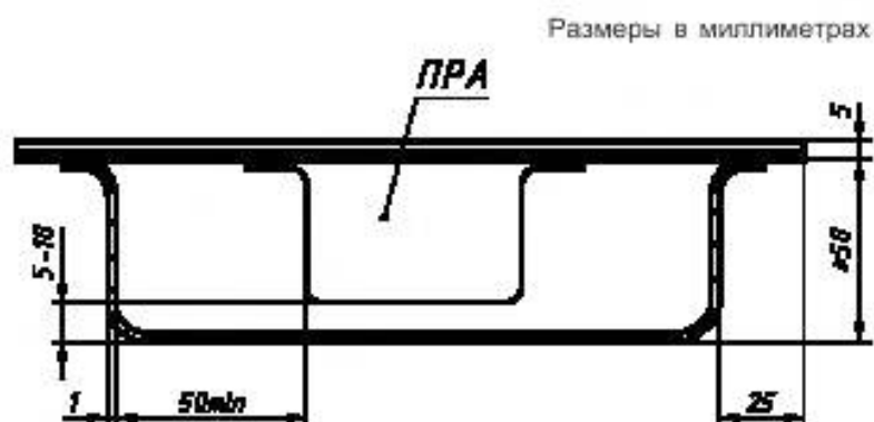
Рисунок 6 — Испытательный корпус для тепловых испытаний ПРА
